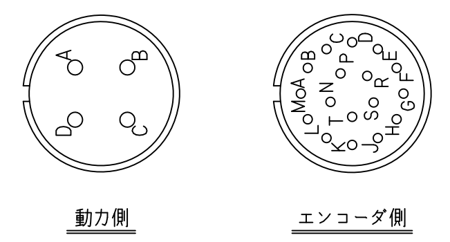
コネクタ向き詳細
