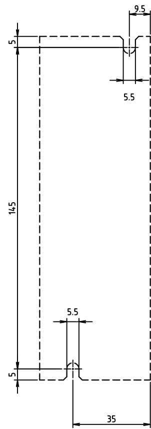
取付穴位置
