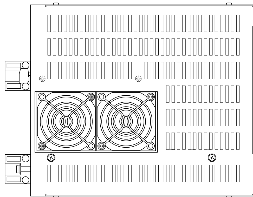
VC II 外形図 拡張I/0付 SE-60450
