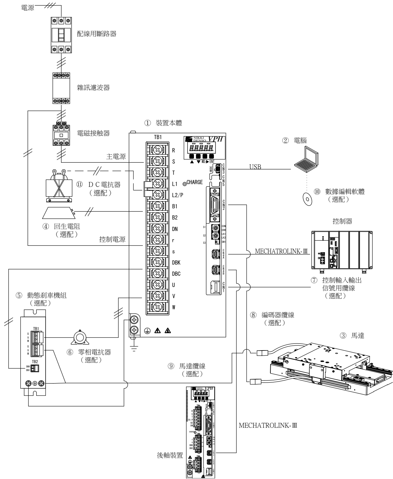
圖1-2 1.5kW級以上VPH HE類型 系統構成
