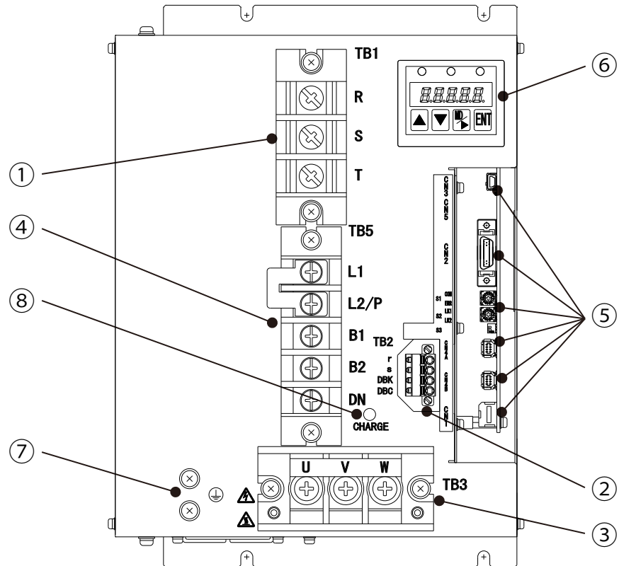
圖13-12 15kW裝置本體正面圖（Type6）
