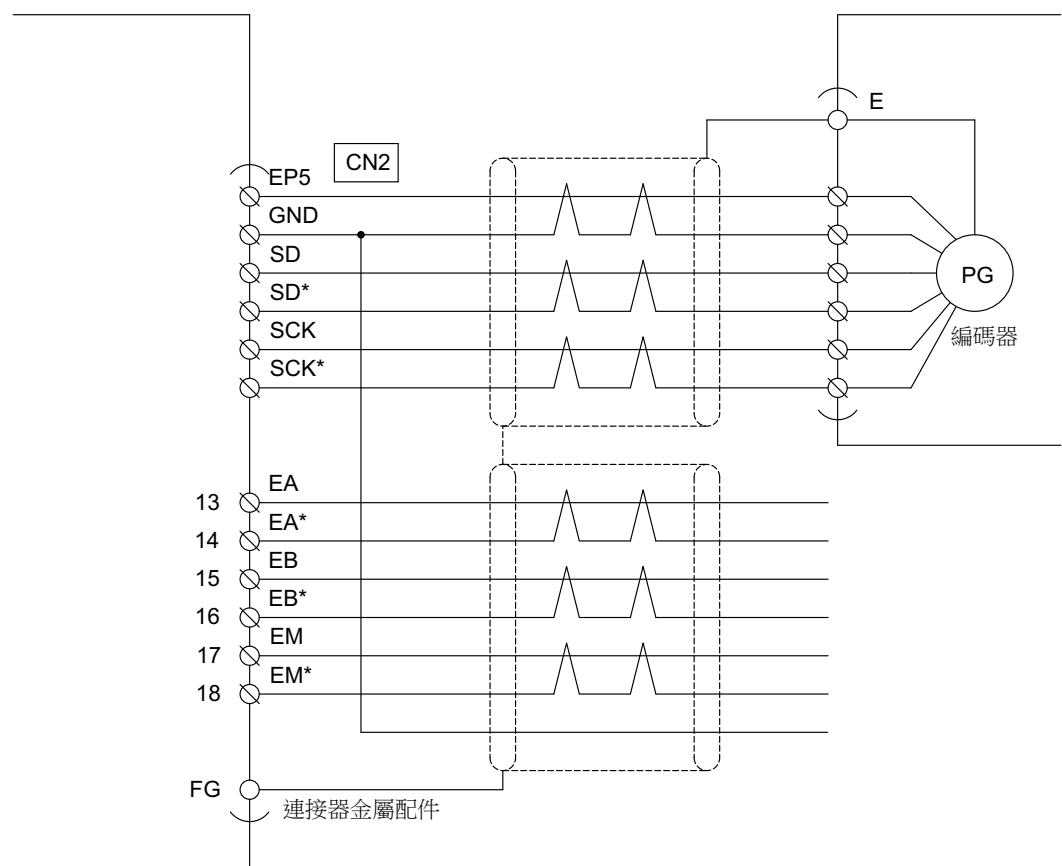
圖3-2 串列編碼器連接圖
