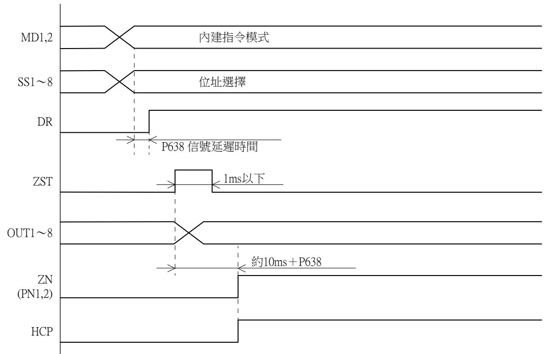
圖5-18 SET ABS 時序圖
