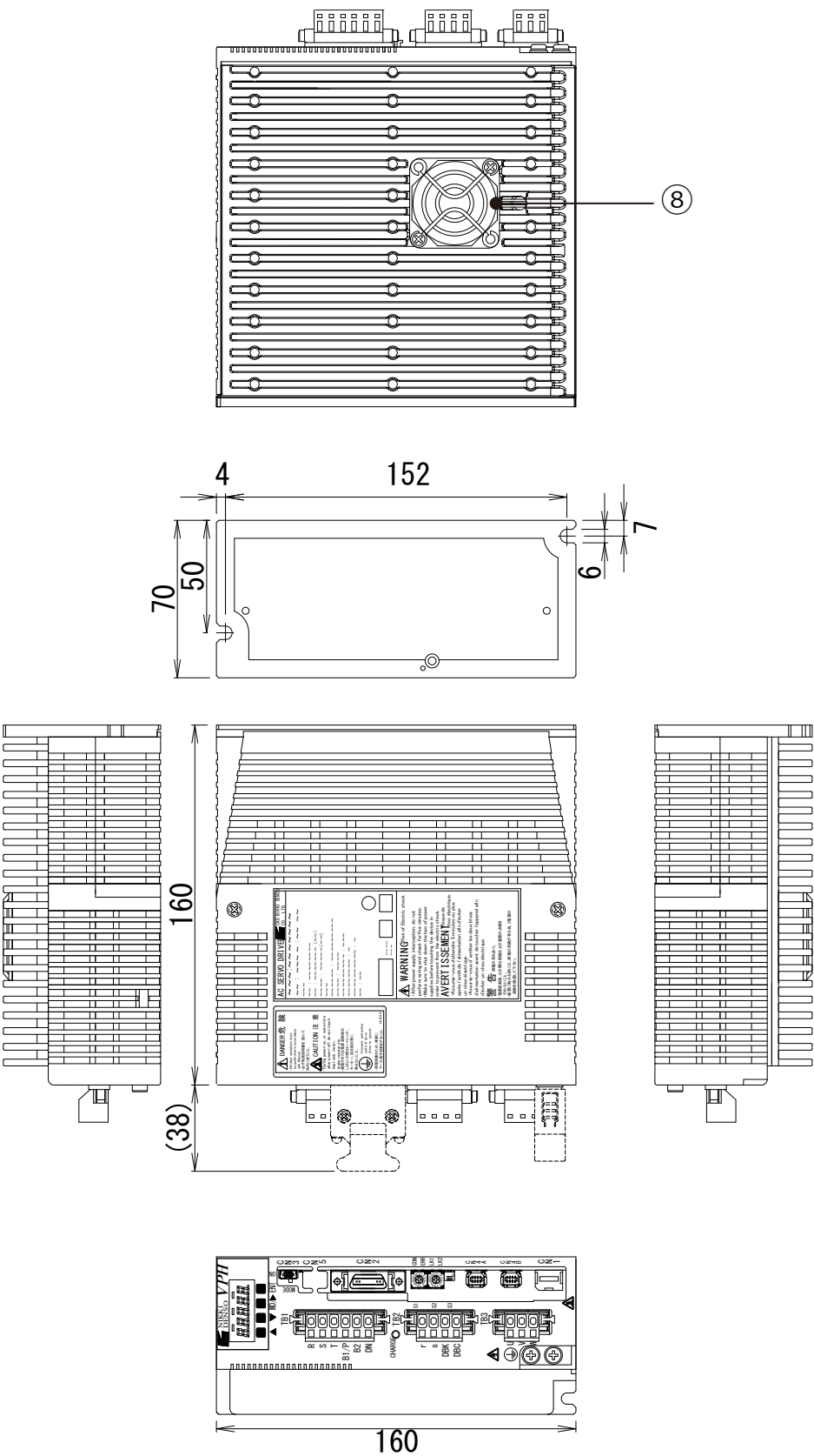
圖13-3 800W裝置本體外形圖（Type2）
