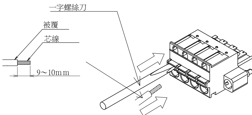
圖2-14 插頭連接器配線圖（200V 7kW,15kW）
