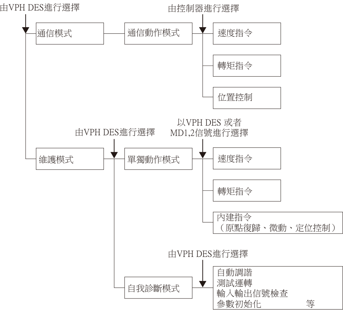
圖1-5 模式構成圖
