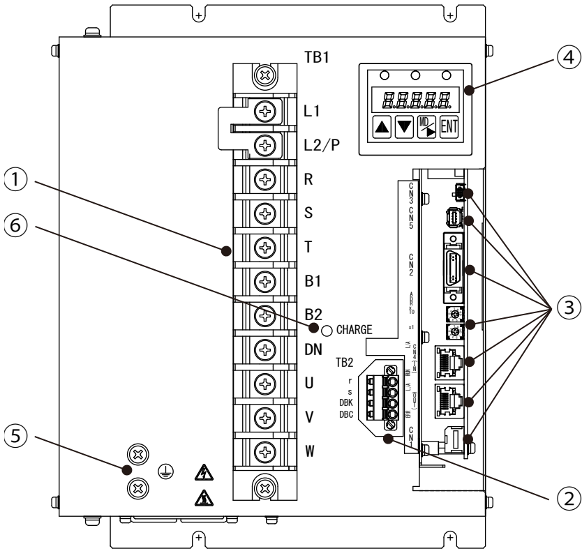
圖13-10 200V 7kW裝置本體正面圖（Type5）
