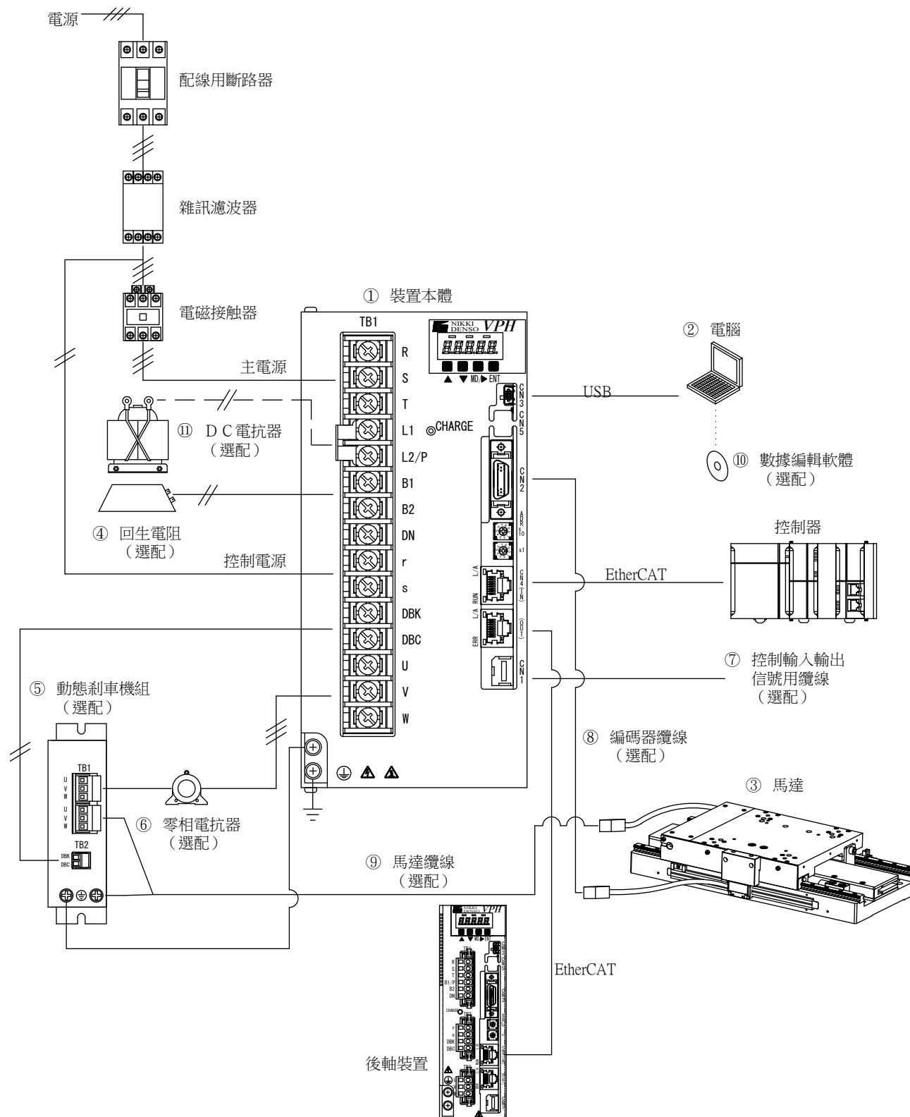
圖1-2 1.5kW級以上VPH HD類型 系統構成
