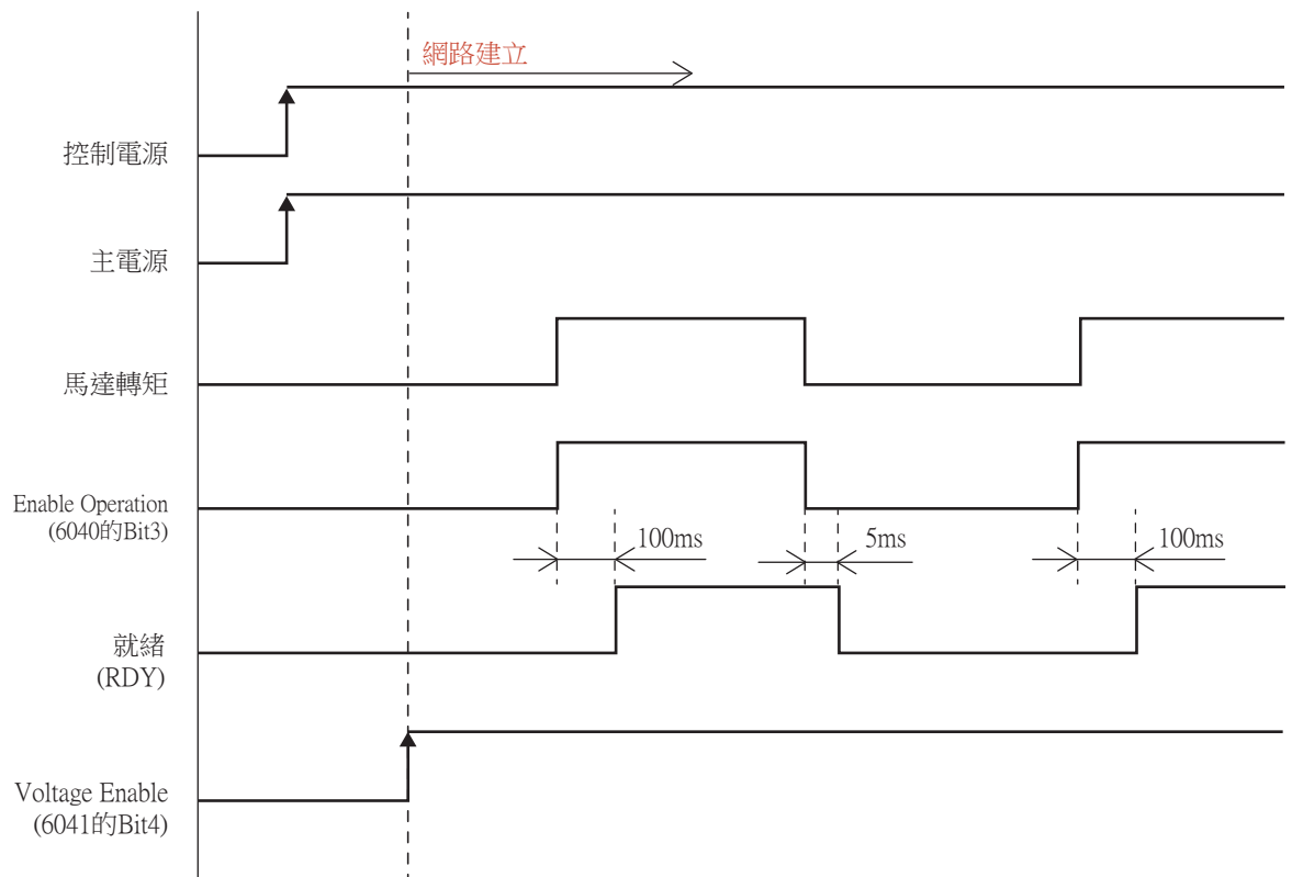
圖2-10 定時圖
