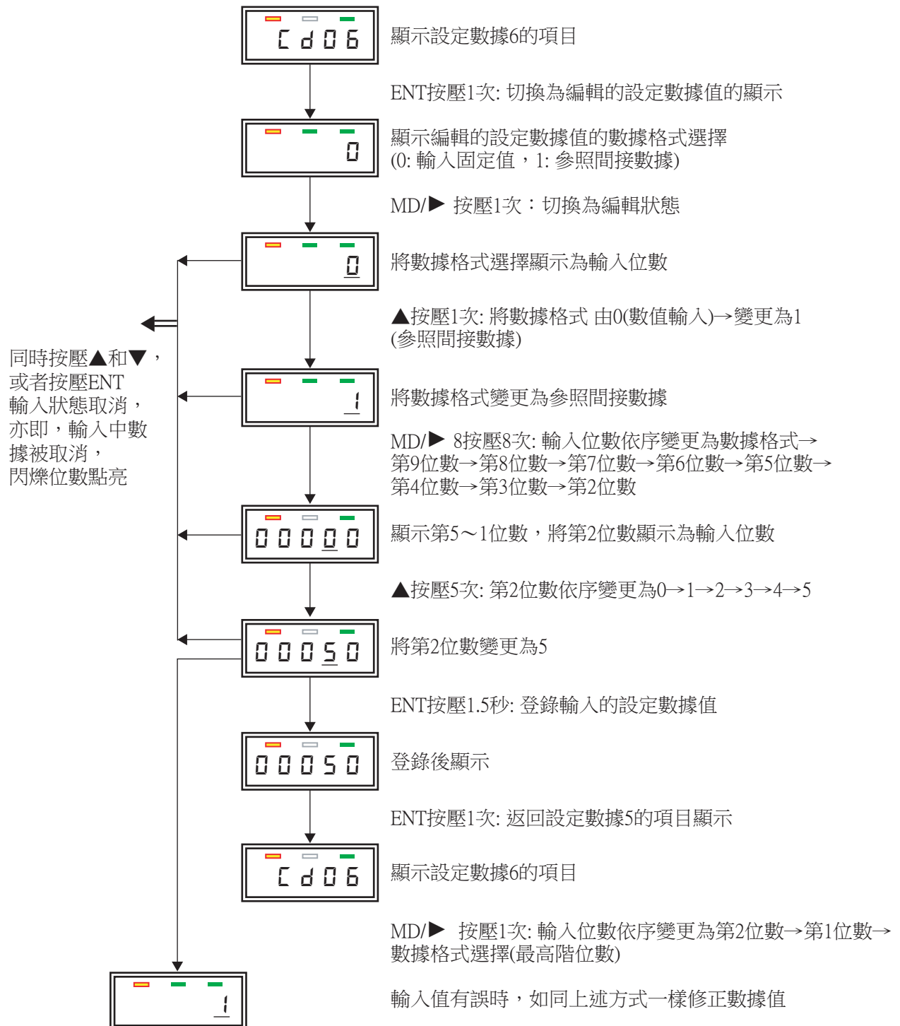
圖12-13 命令編輯範例 (4/4)
