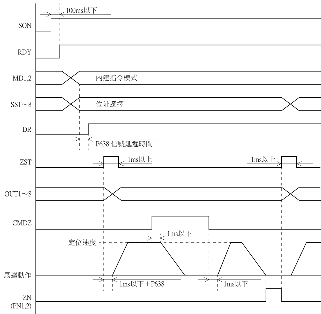
圖5-18 POS命令時序圖
