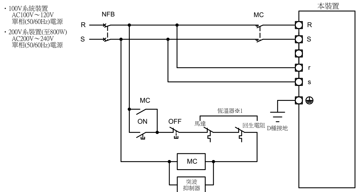
圖2-9 單相電源時具代表性的電源迴路
