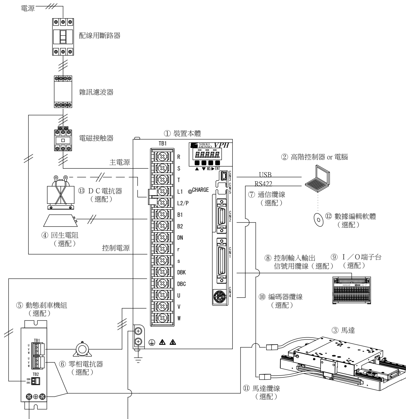
圖1-2 1.5kW級以上VPH HA類型 系統構成
