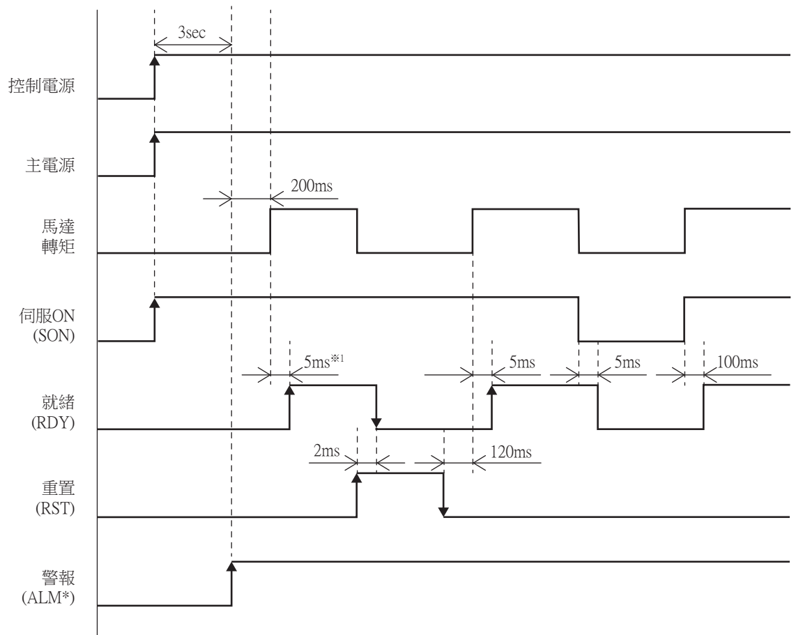
圖2-10 定時圖
