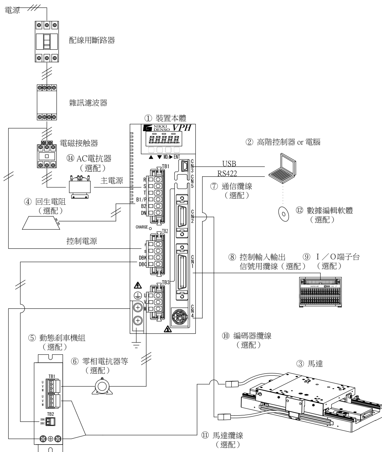
圖1-1 800W級以下VPH HA類型 系統構成
