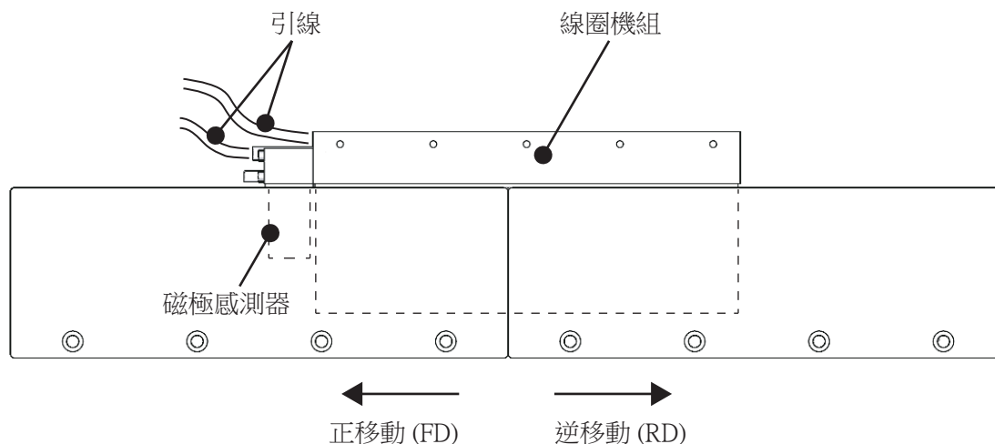
圖4-1 線圈機組與磁極感測器的動作方向
