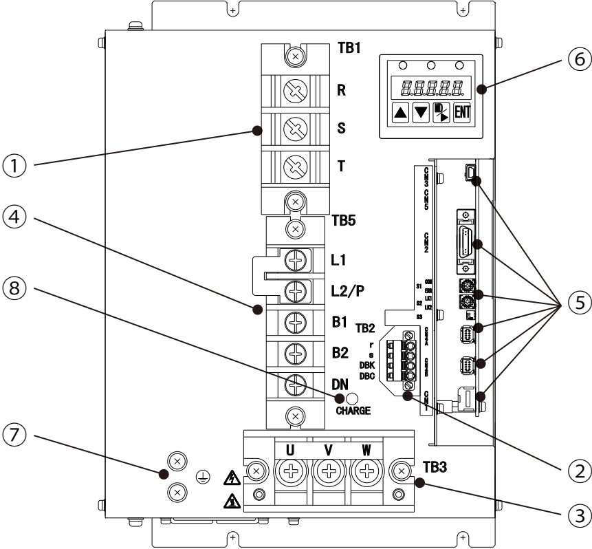
圖13-12 15kW裝置本體正面圖（Type6）
