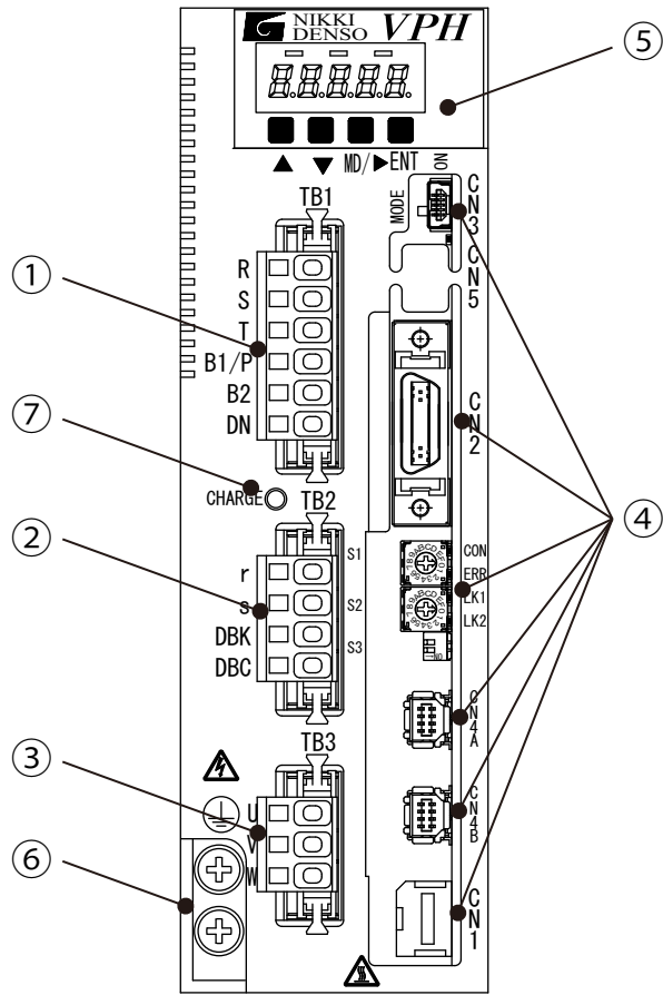
圖13-2 400W以下裝置本體正面圖（Type1）
