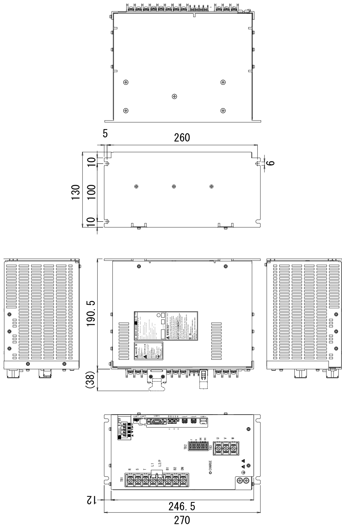
圖13-7 3.3kW裝置本體外形圖（Type4）
