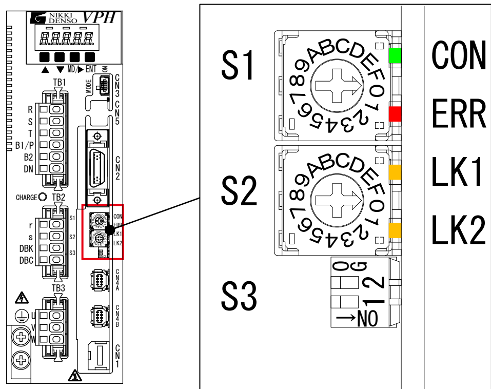
圖1-3 站位址設定
