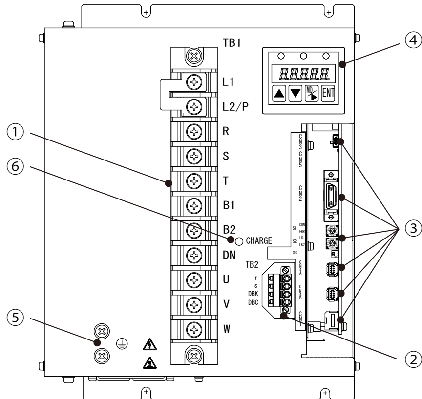
圖13-10 200V 7kW裝置本體正面圖（Type5）
