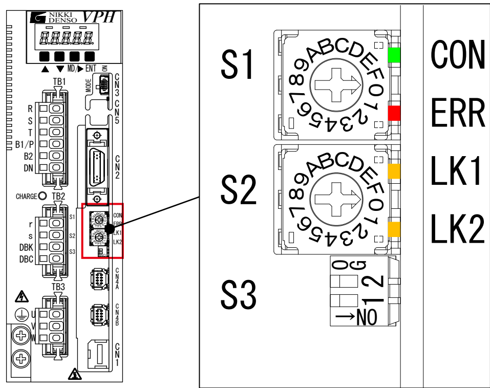
圖1-4 通信狀態顯示LED外觀
