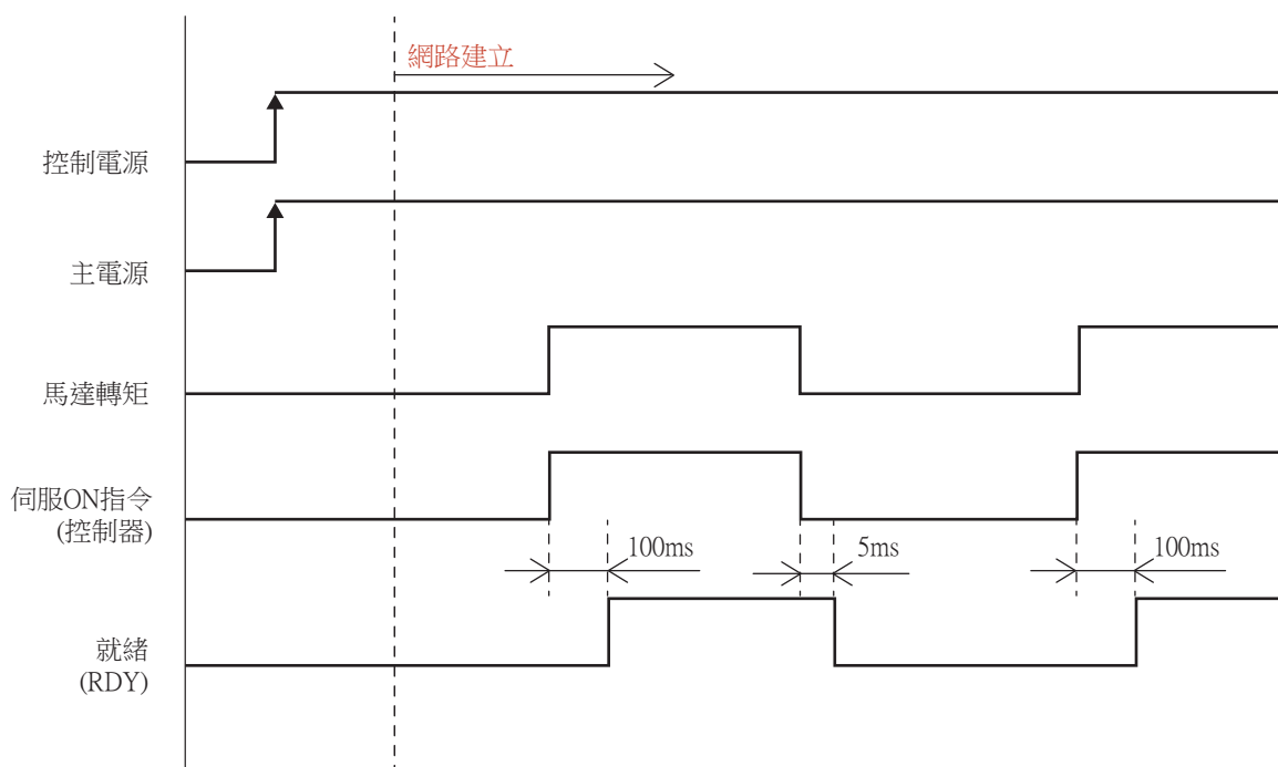
圖2-11 定時圖
