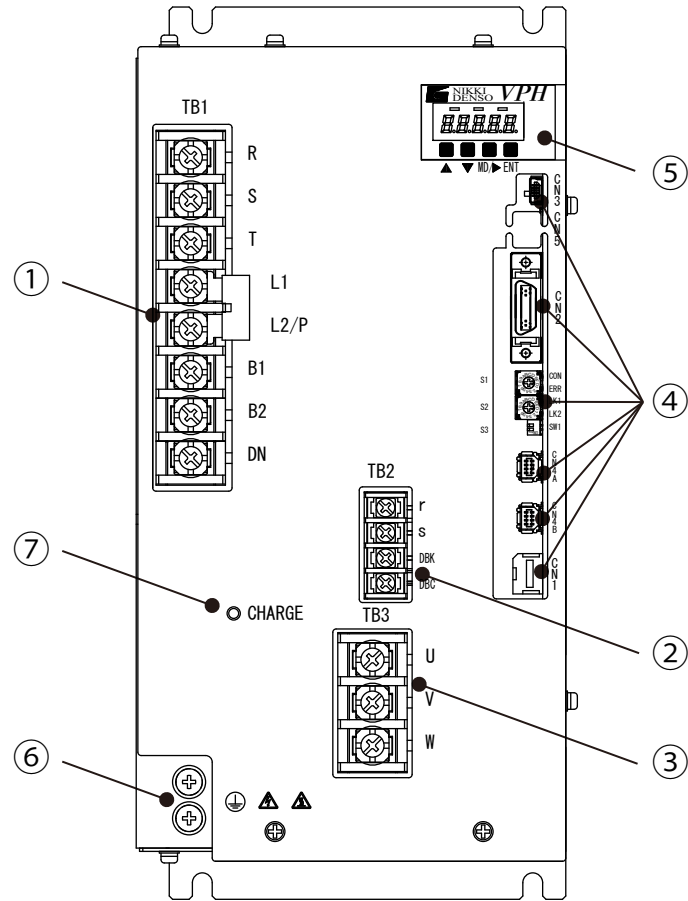
圖13-8 3.3kW裝置本體正面圖（Type4）
