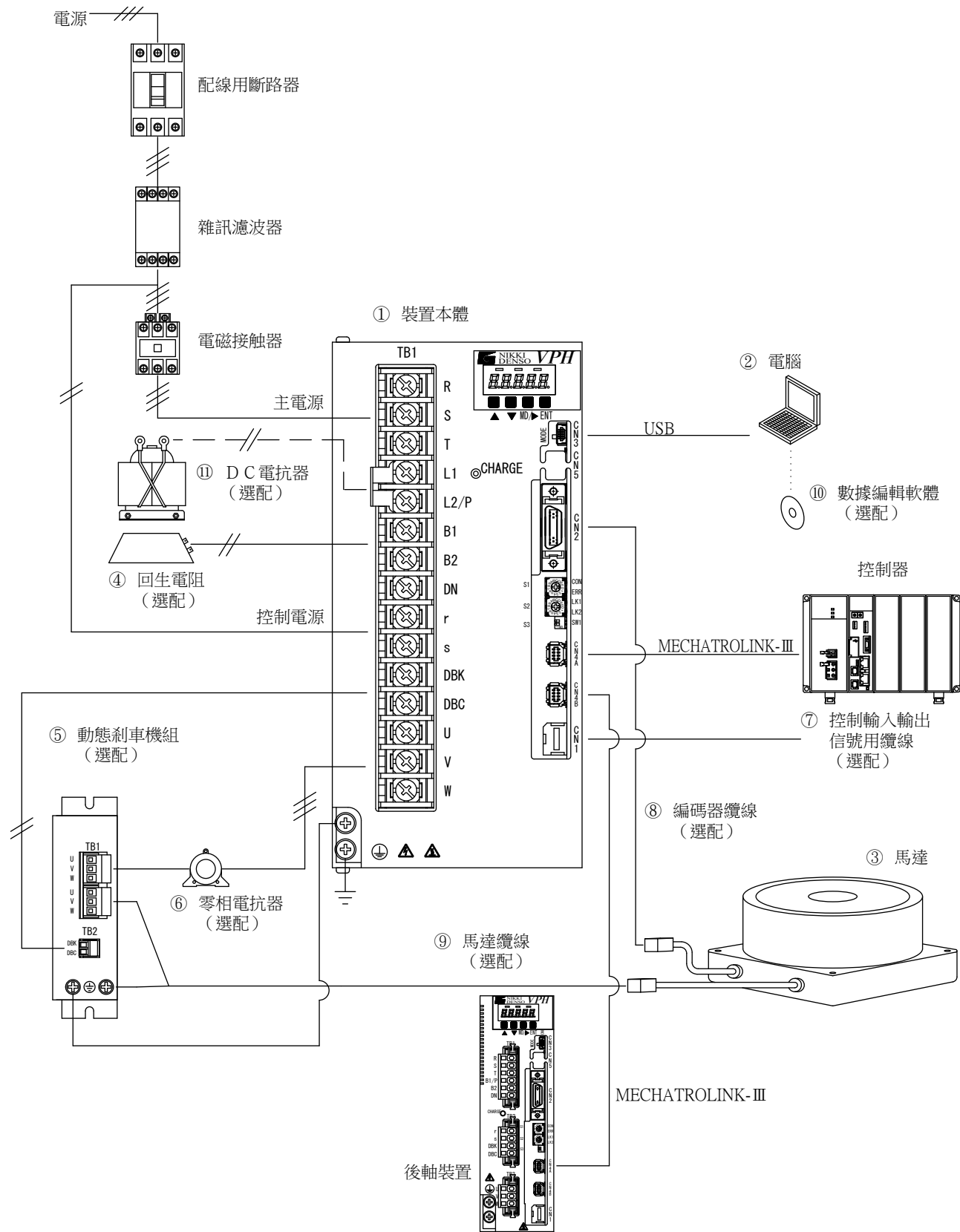
圖1-2 1.5kW級以上VPH HE類型 系統構成
