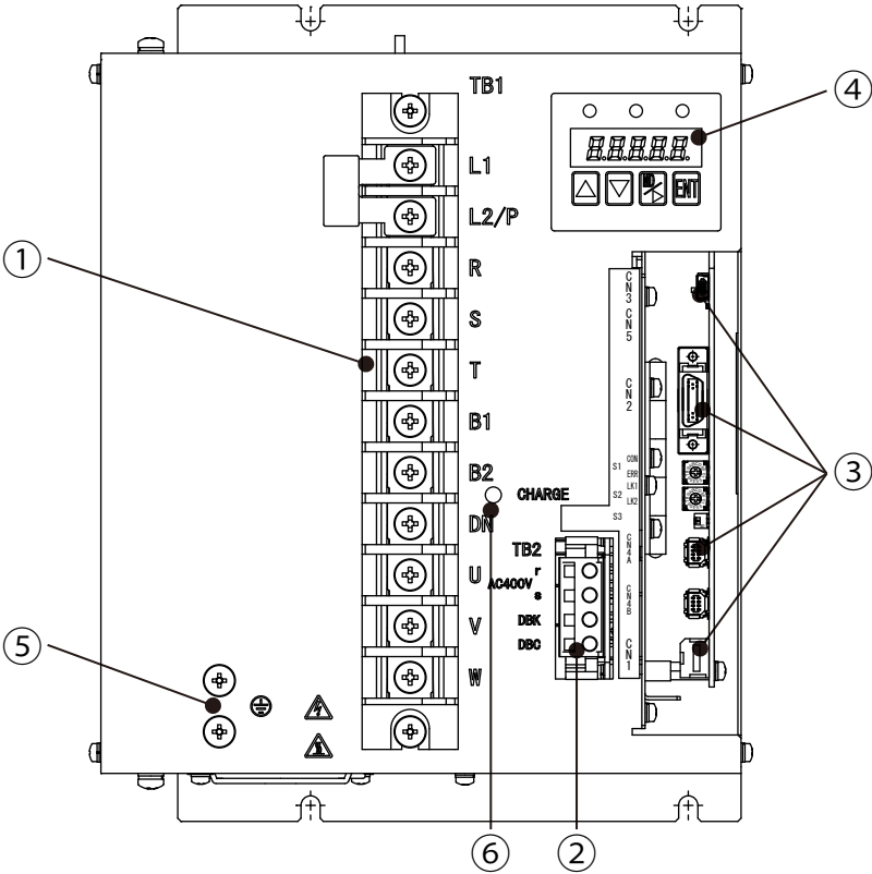
圖13-14 400V 7kW裝置本體正面圖（Type7）
