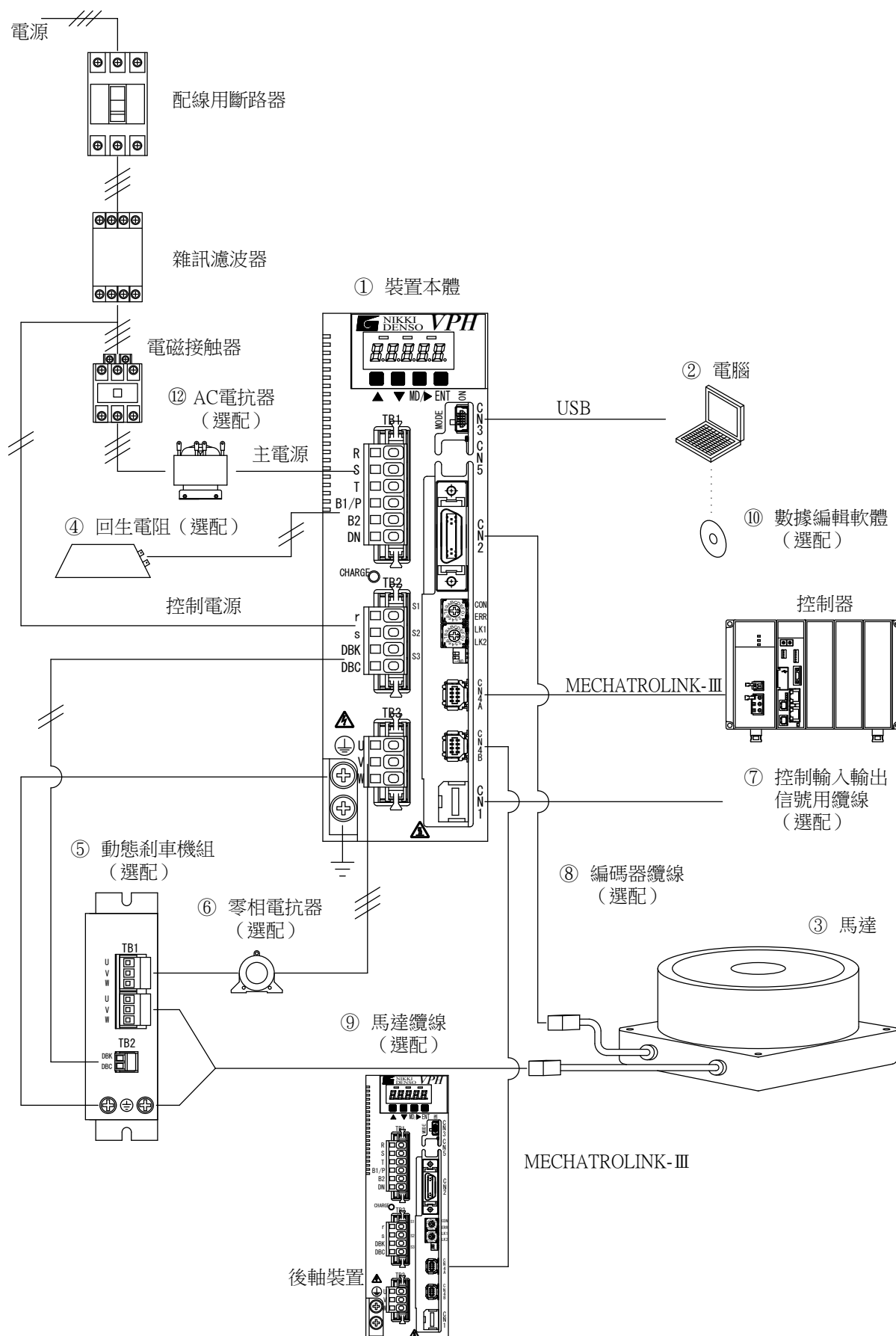
圖 1-1 800W 級以下 VPH HE 類型 系統構成
