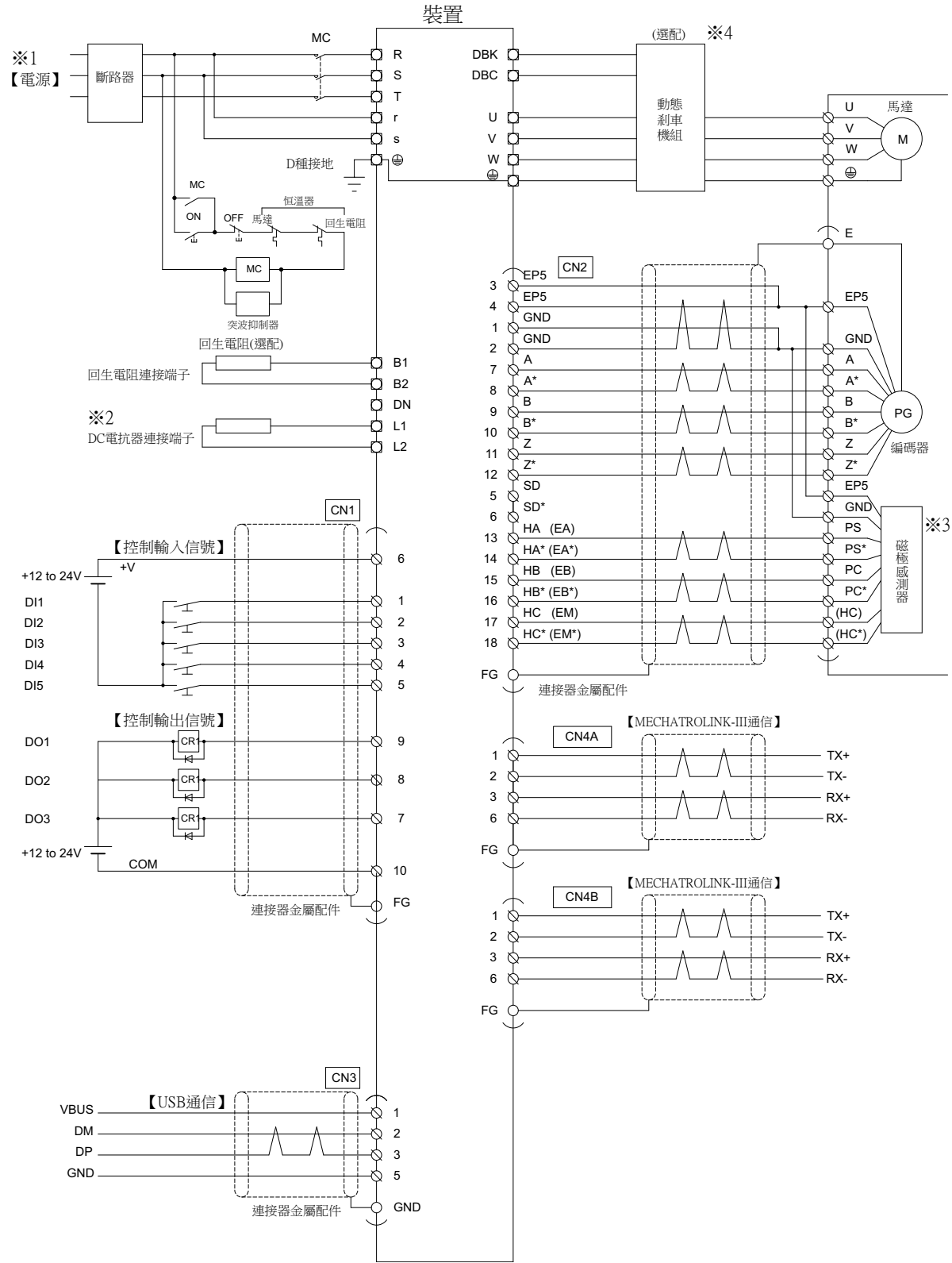
圖3-1 外部連接圖
