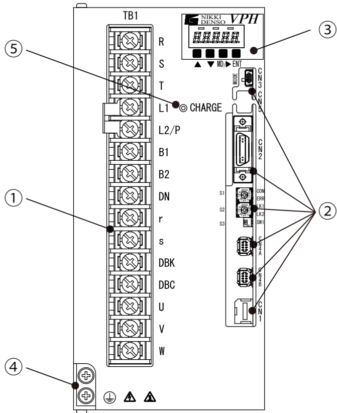
圖13-6 1.5kW、2.2kW裝置本體正面圖（Type3）
