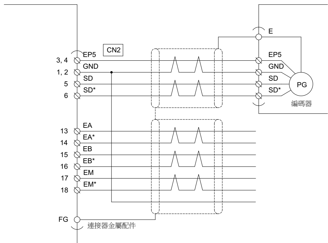
圖3-2 串列編碼器連接圖
