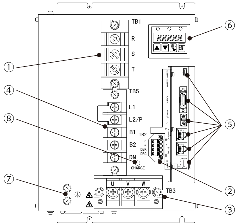
圖13-12 15kW裝置本體正面圖（Type6）
