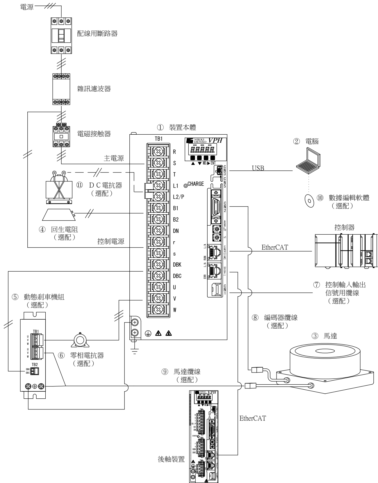
圖1-2 1.5kW級以上VPH HD類型 系統構成
