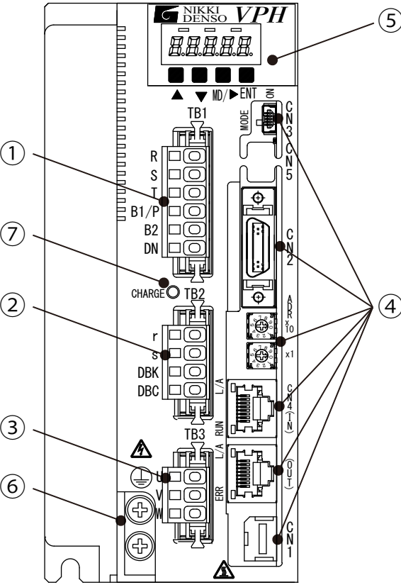
圖13-4 800W裝置本體正面圖（Type2）
