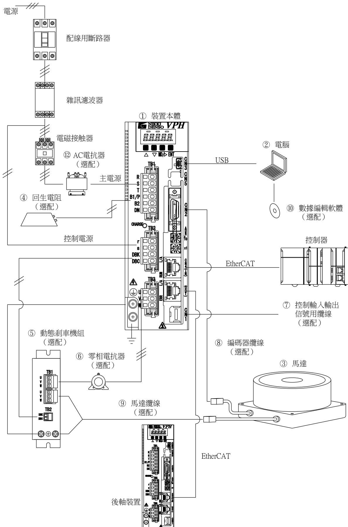
圖 1-1 800W 級以下 VPH HD 類型 系統構成
