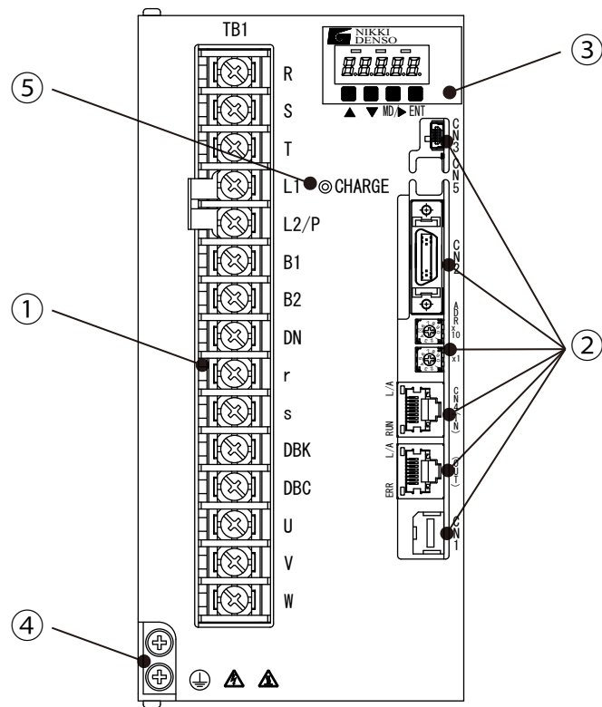
圖13-6 1.5kW、2.2kW裝置本體正面圖（Type3）
