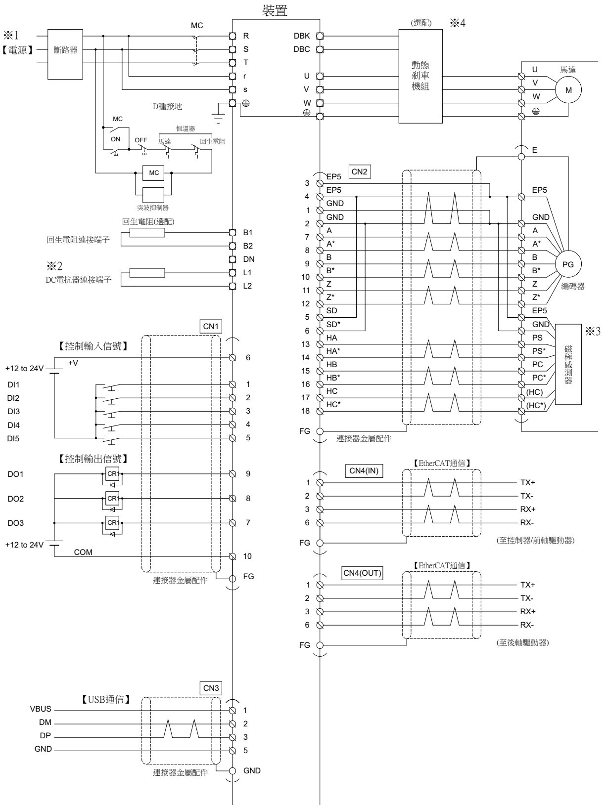
圖3-1 外部連接圖
