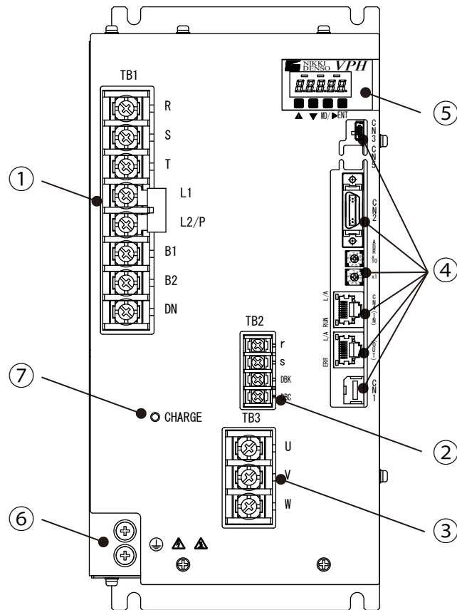
圖13-8 3.3kW裝置本體正面圖（Type4）
