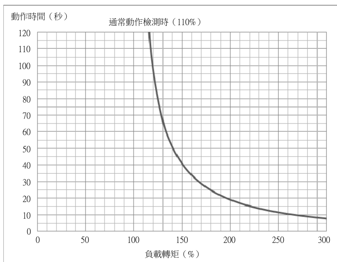
圖8-1 負載轉矩與檢測時間的關係
