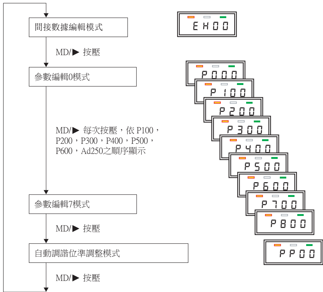
圖12-4 參數編輯模式的構成和轉變
