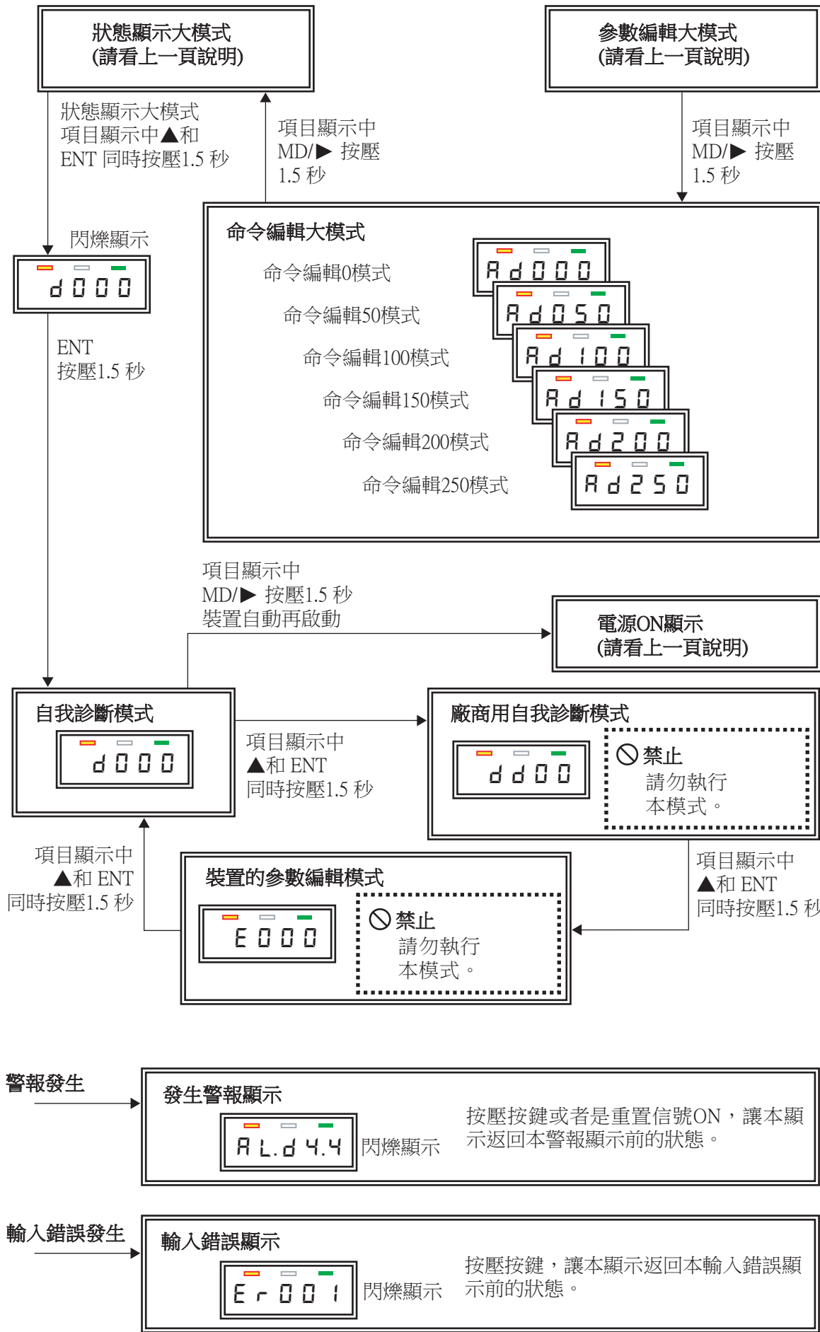
圖12-3 操作模式的構成和轉變（2/2）
