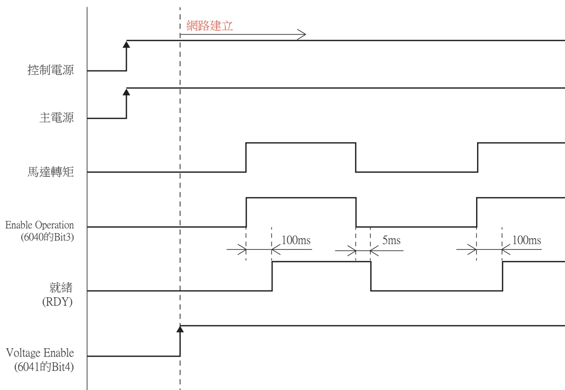
圖2-11 定時圖
