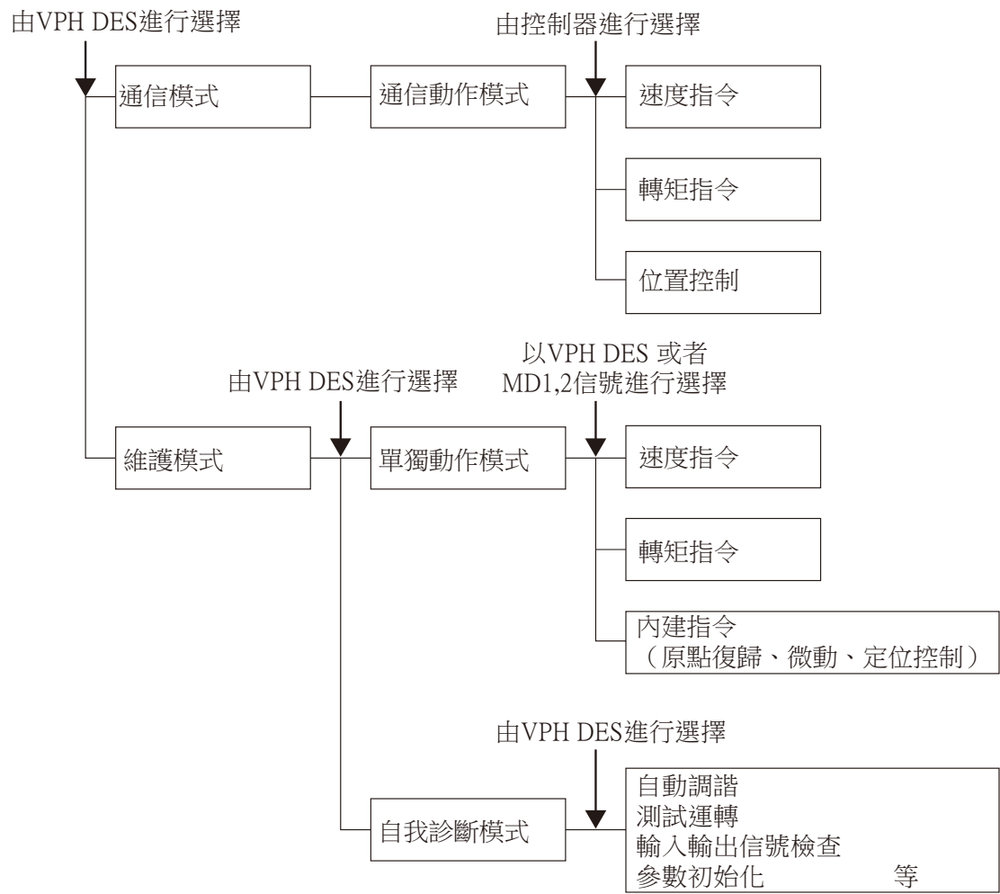
圖1-5 模式構成圖
