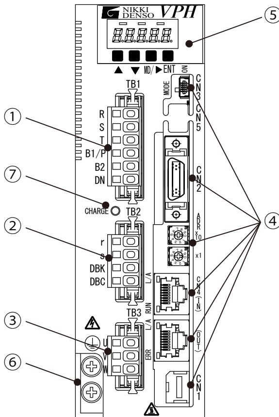
圖13-2 400W以下裝置本體正面圖 (Type1)
