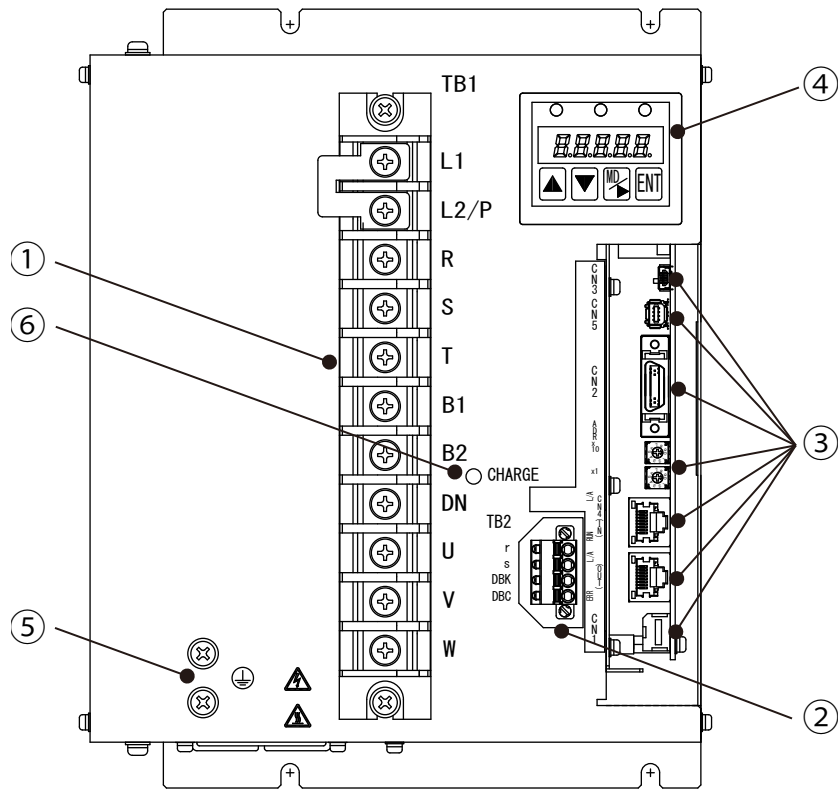
圖13-10 200V 7kW裝置本體正面圖（Type5）
