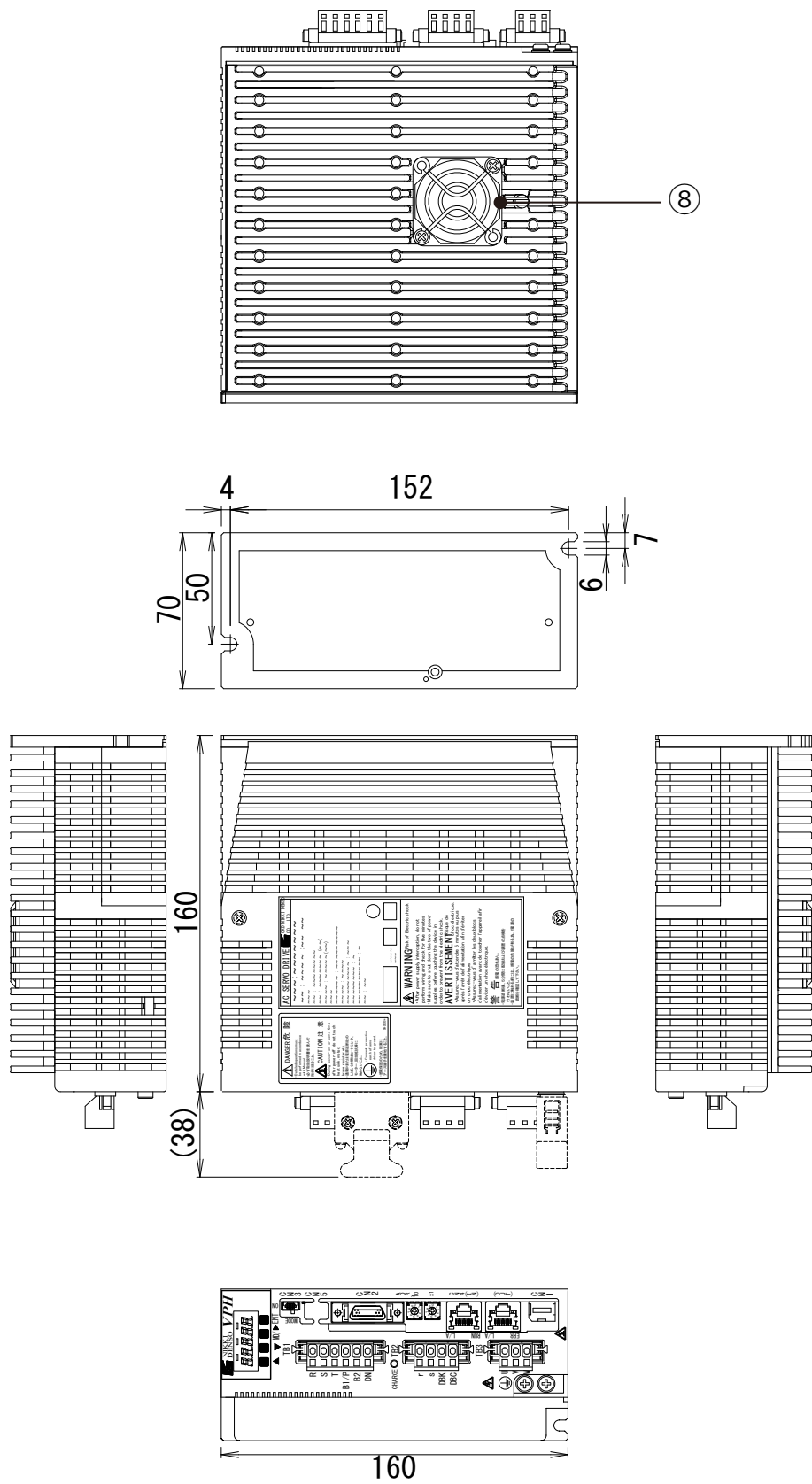
圖13-3 800W裝置本體外形圖（Type2）
