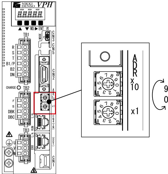
圖1-3 節點位址選擇開關
