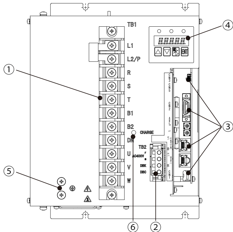
圖13-14 400V 7kW裝置本體正面圖（Type7）
