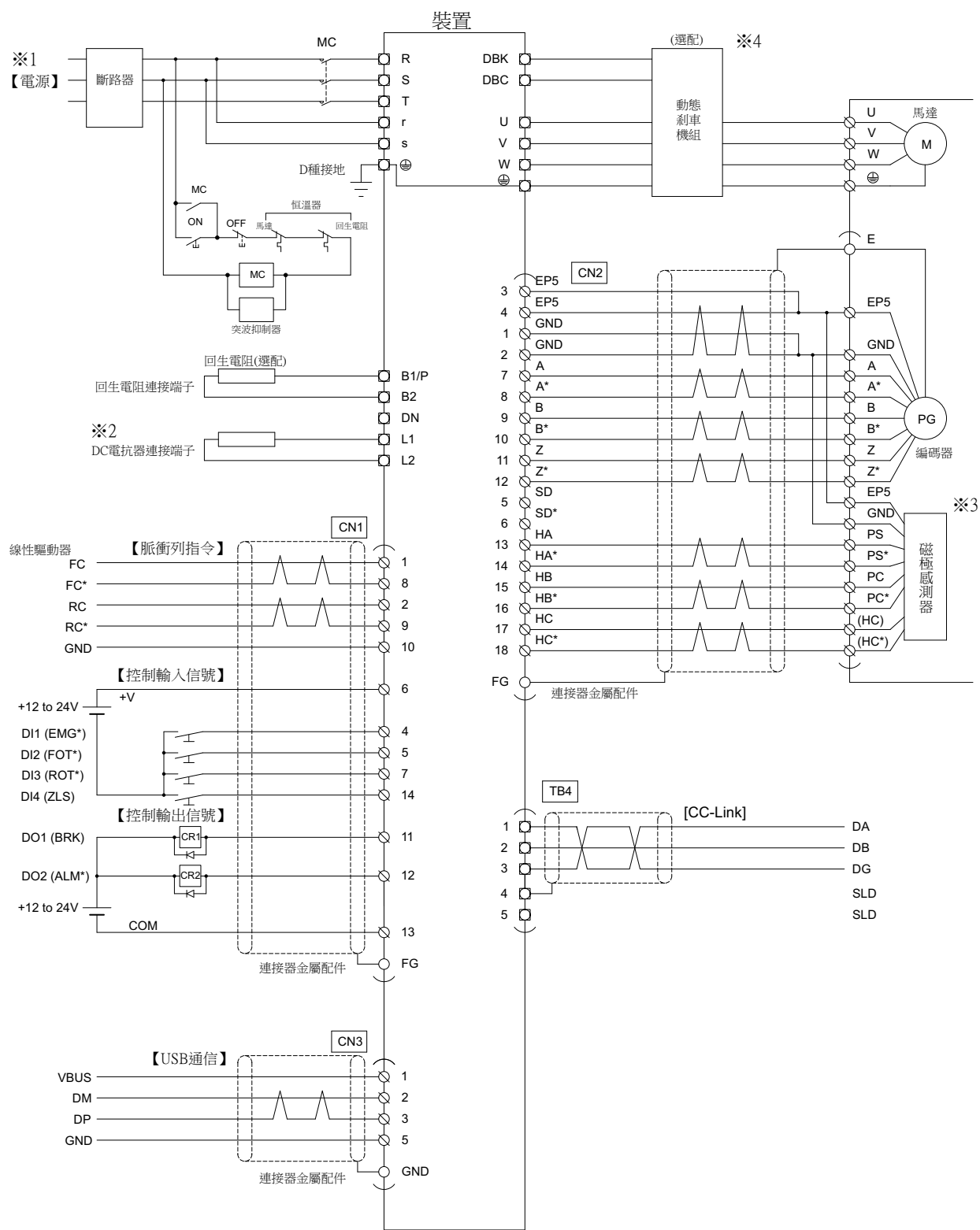
圖3-1 外部連接圖
