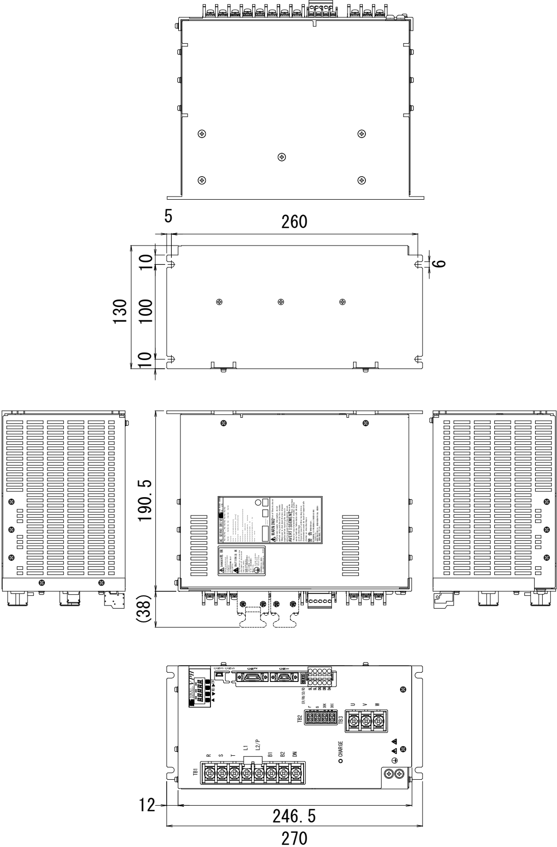
圖13-7 3.3kW裝置本體外形圖（Type4）
