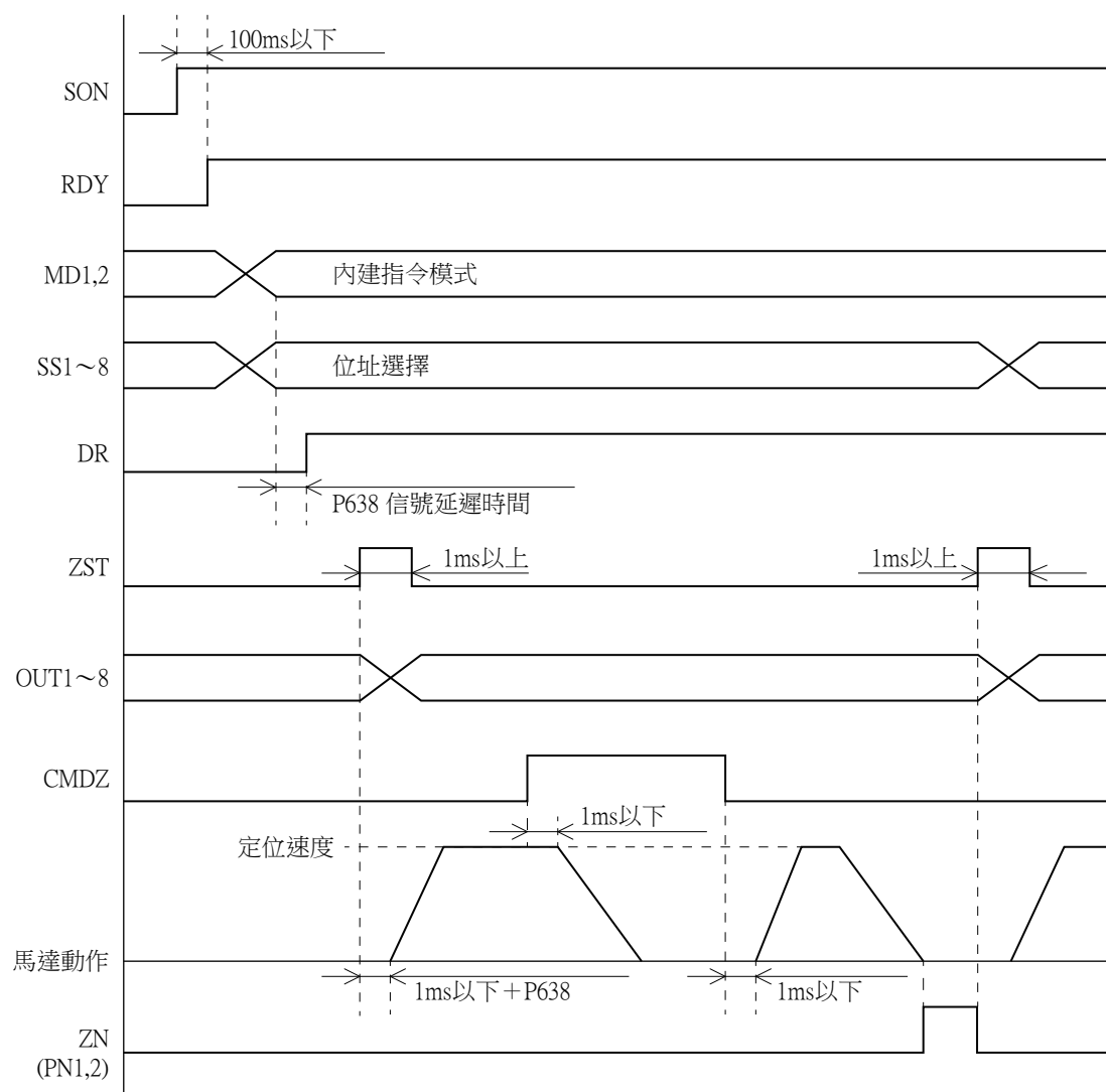
圖5-21 INDX命令時序圖
