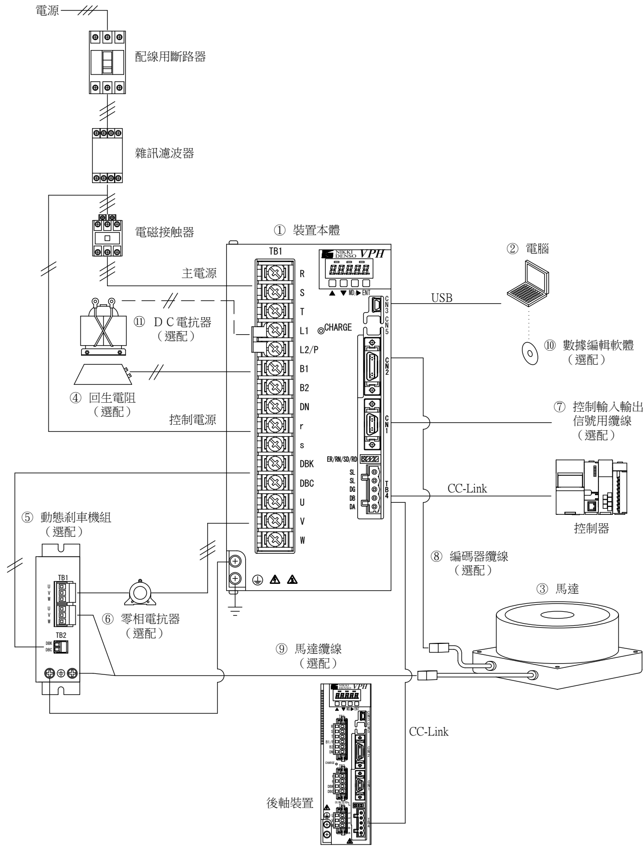
圖1-2 1.5kW級以上VPH HC類型 系統構成
