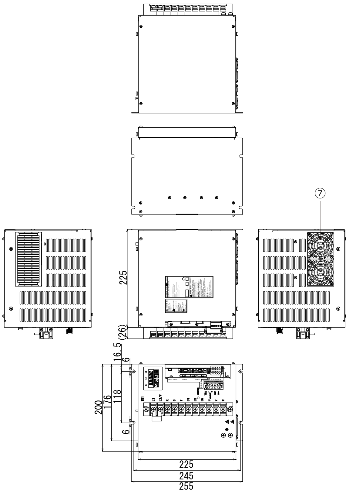
圖13-13 400V 7kW裝置本體外形圖 (Type7)
