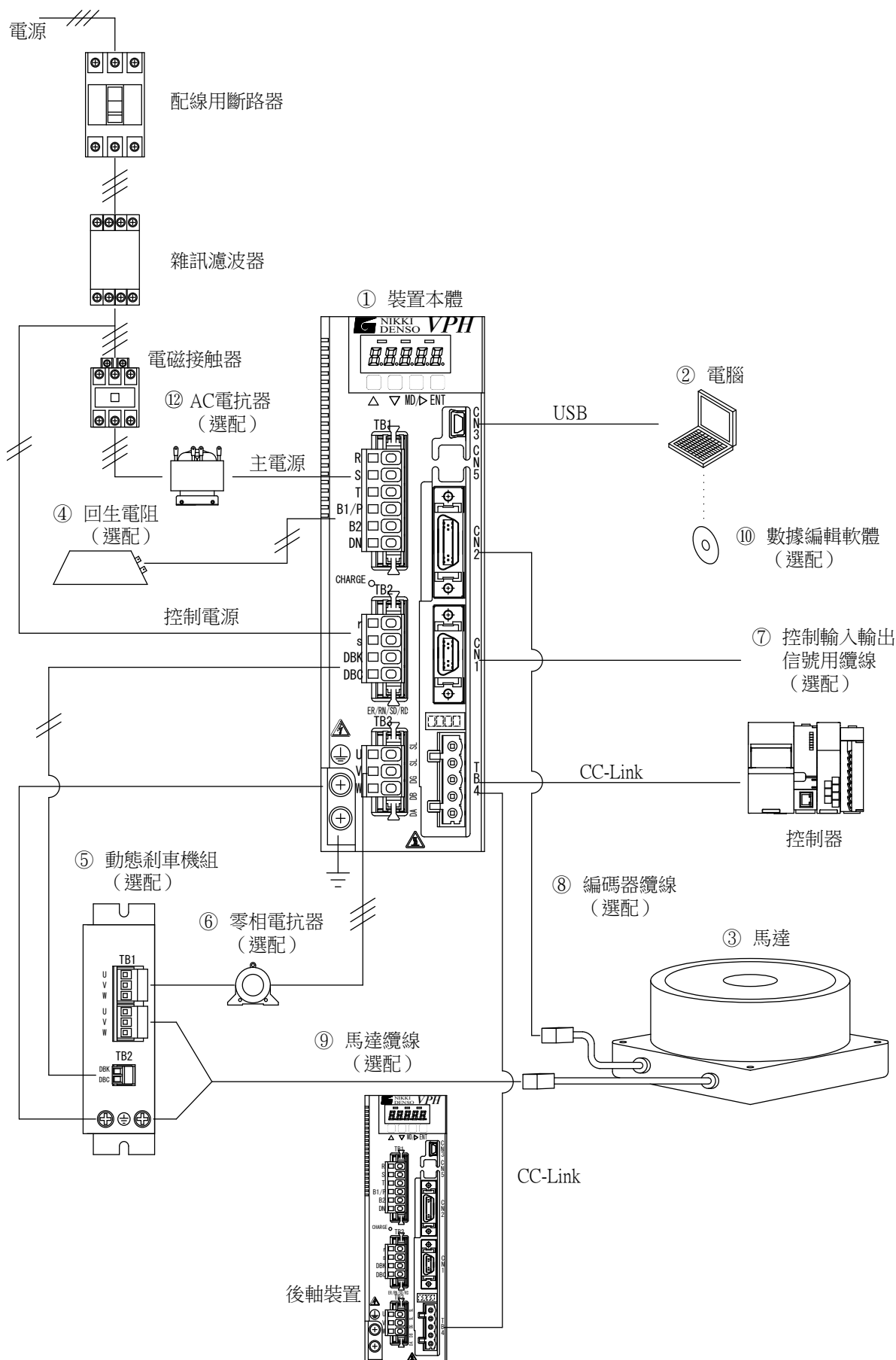
圖 1-1 800W 級以下 VPH HC 類型 系統構成
