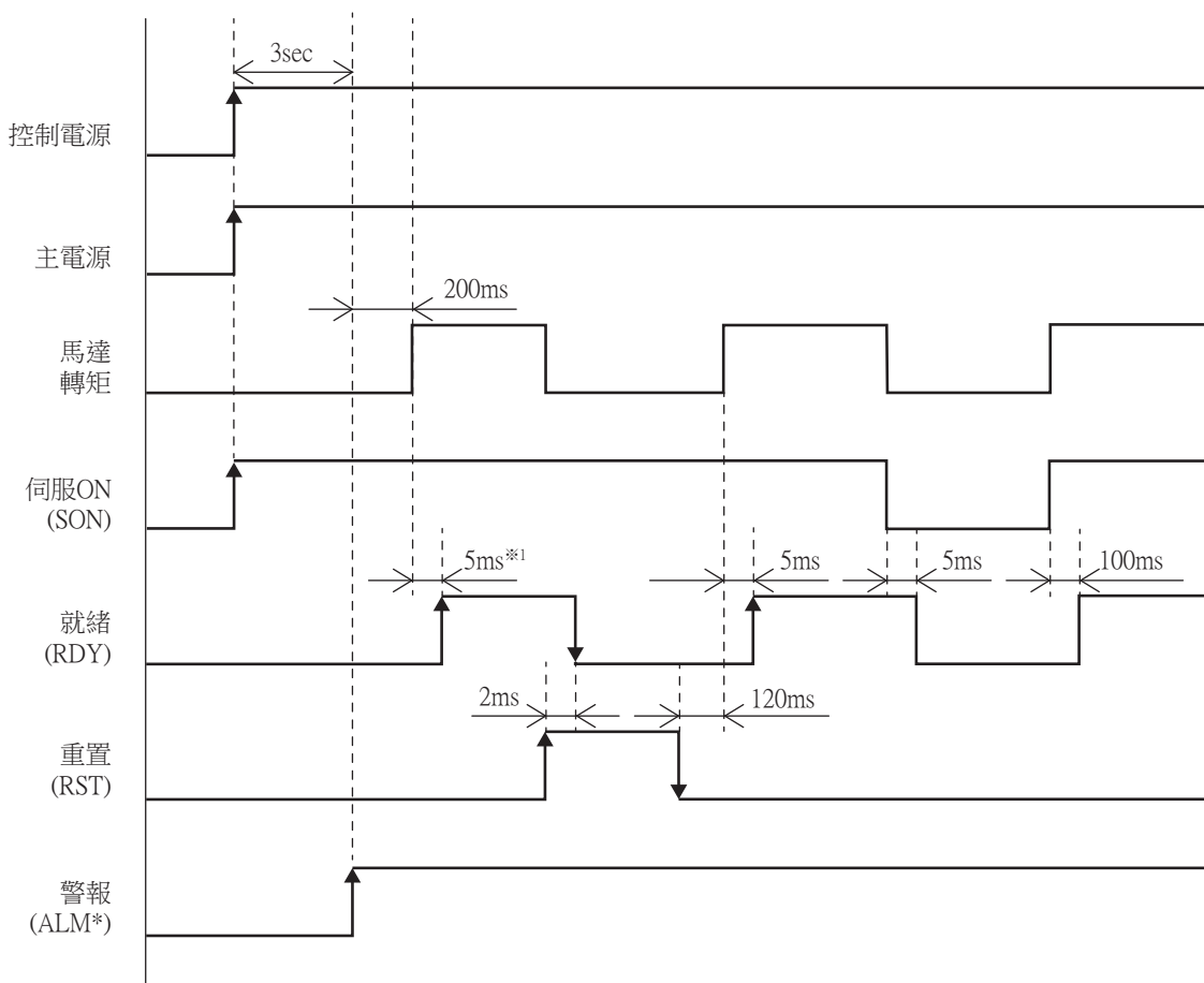
圖2-11 定時圖
