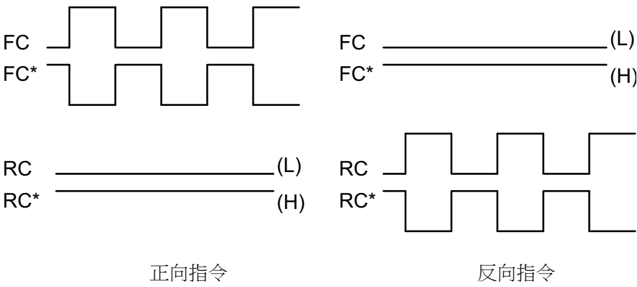
圖3-4 方向別脈衝
