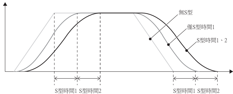
圖5-16 S型加減速動作例
