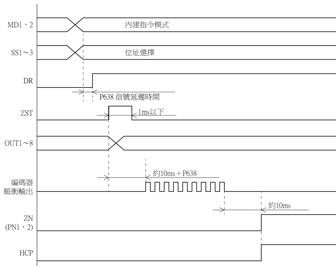
圖5-30 OUT POS 時序圖
