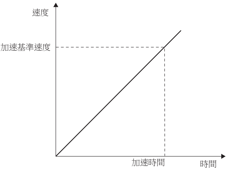
圖5-4 速度指令模式時的加速基準速度與加速時間的關係
