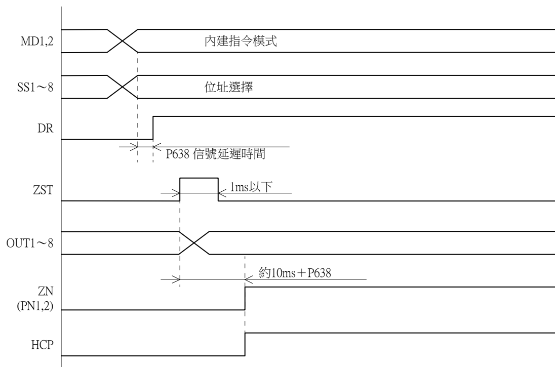
圖5-28 SET ABS 時序圖
