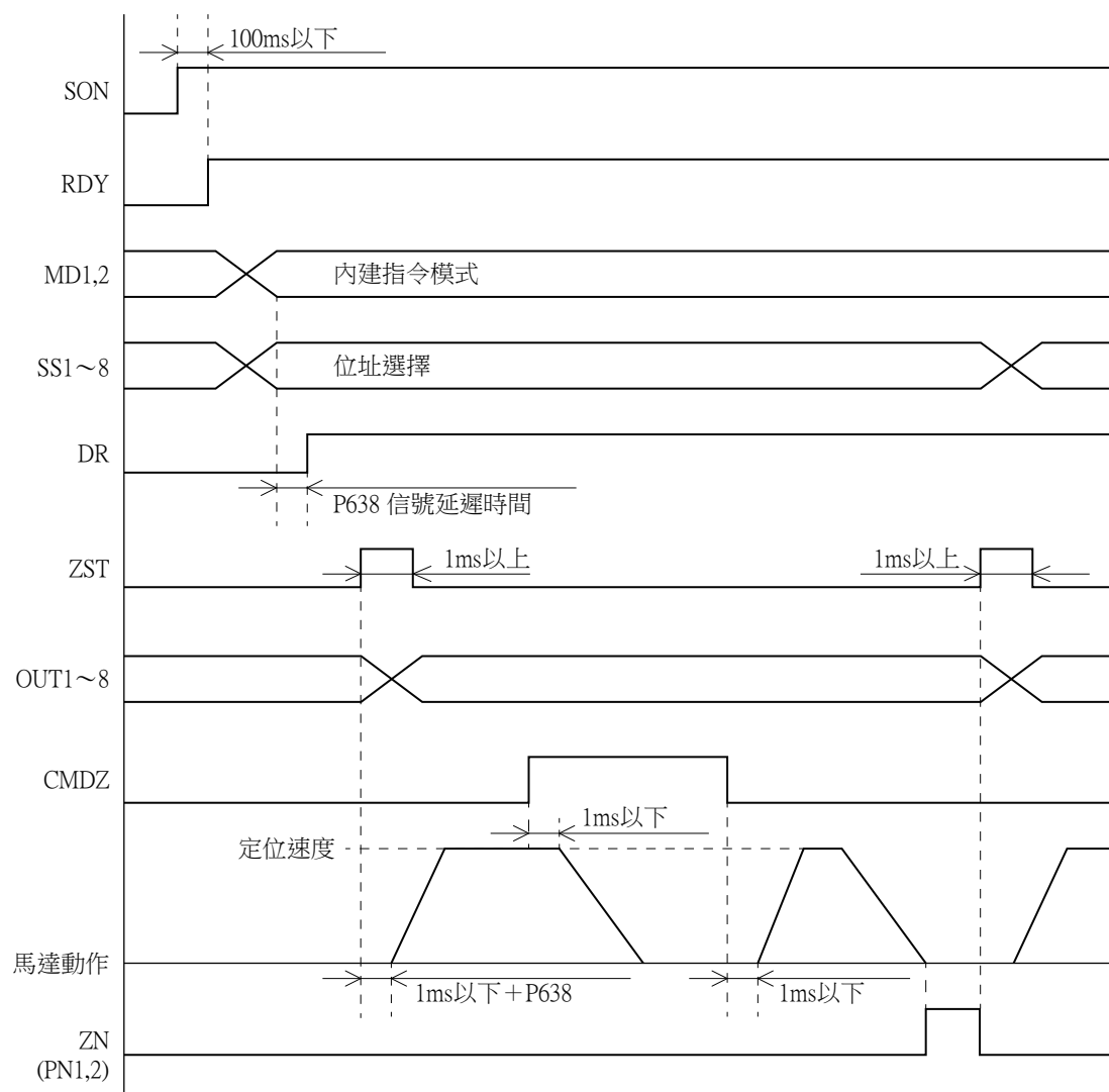
圖5-31 INDX命令時序圖
