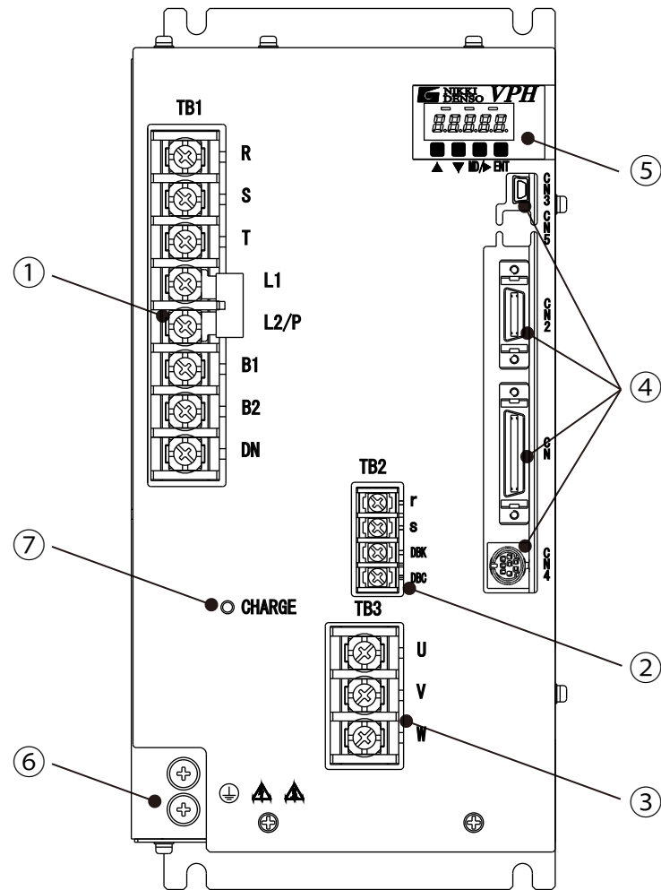
圖13-8 3.3kW裝置本體正面圖（Type4）
