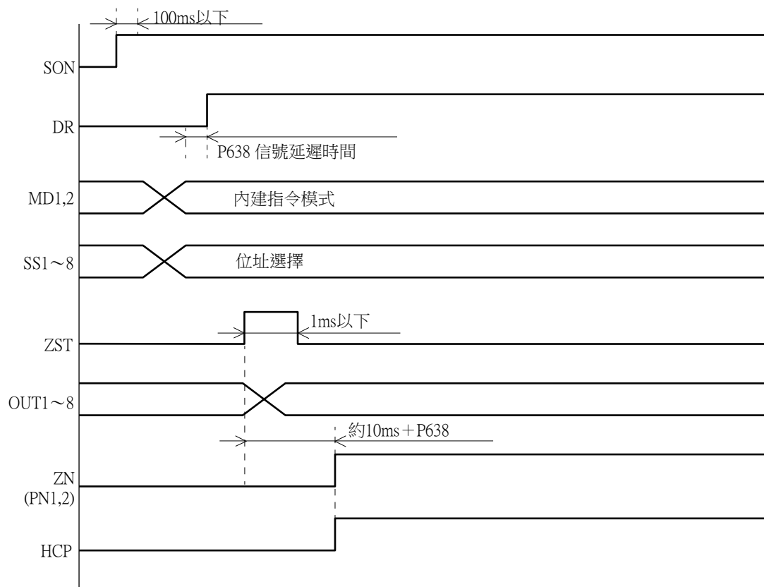
圖5-23 STOP HOME 時序圖
