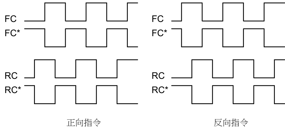
圖3-4 90°相位差信號
