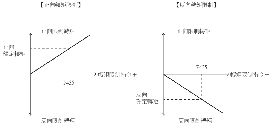
圖5-17 藉由類比轉矩指令的轉矩限制
