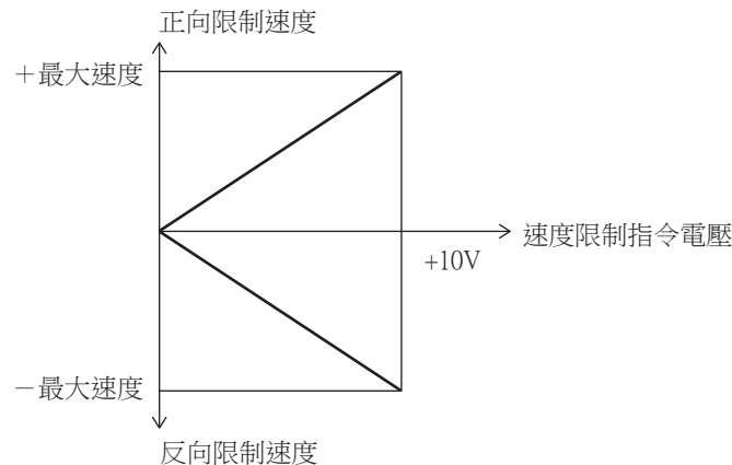
圖5-10 藉由類比速度指令的速度限制
