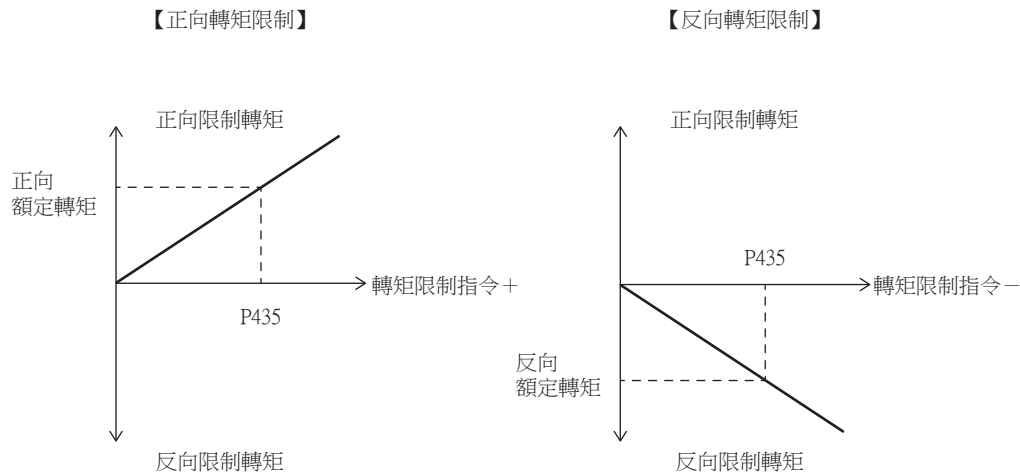
圖5-13 藉由類比轉矩指令的轉矩限制
