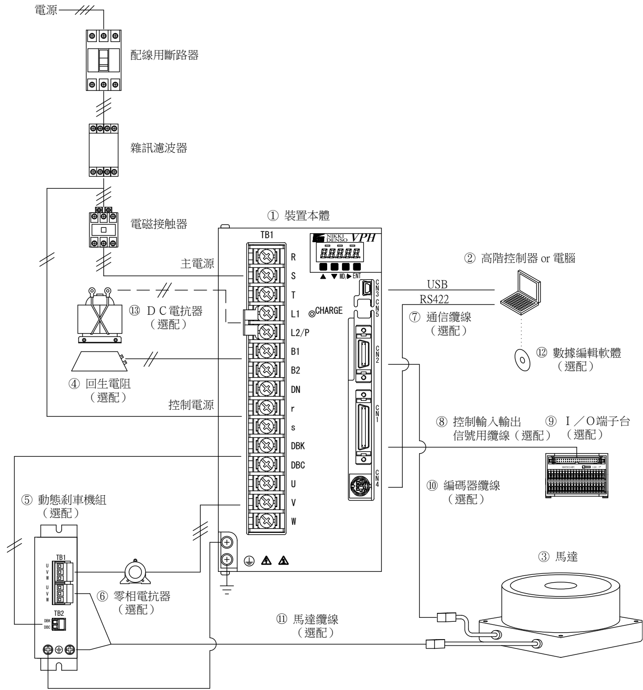
圖1-2 1.5kW級以上VPH HA類型 系統構成
