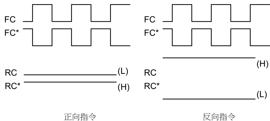
圖3-6 方向信號 + 進給脈衝
