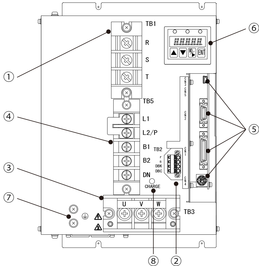
圖13-12 15kW裝置本體正面圖（Type6）
