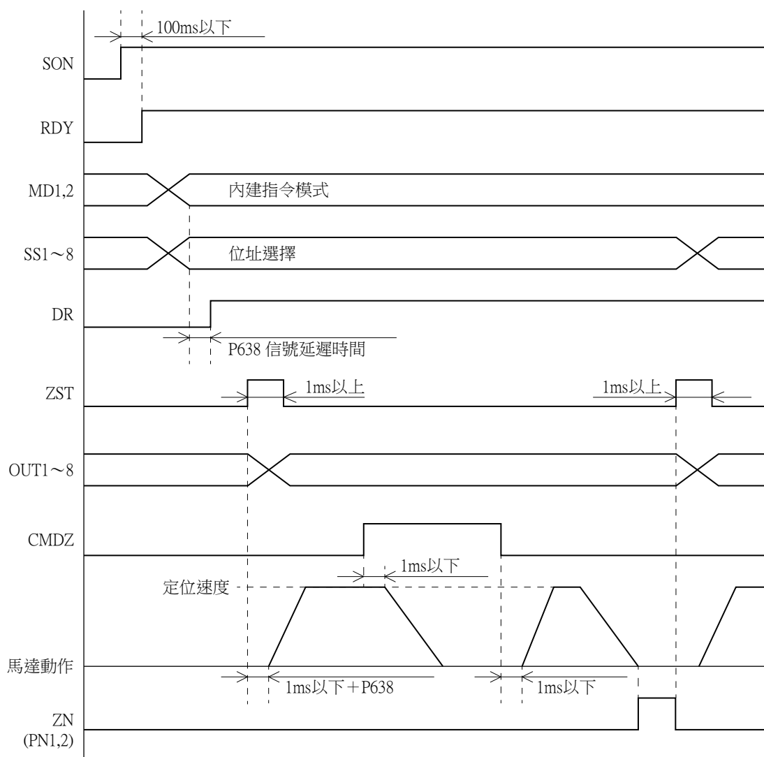
圖5-18 POS命令時序圖
