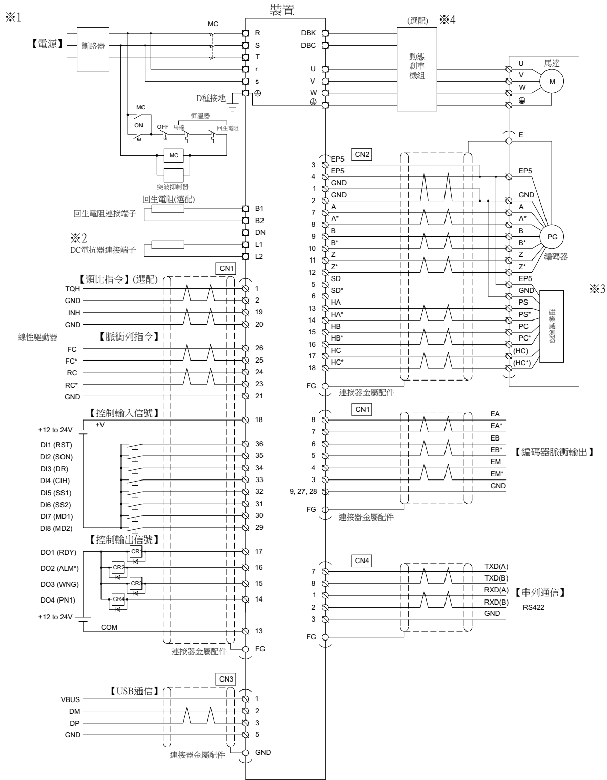
圖3-1 外部連接圖
