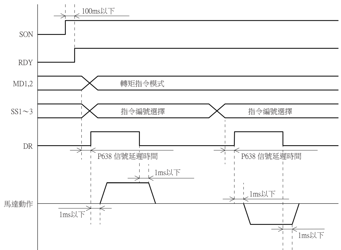
圖5-8 內部轉矩指令時序圖
