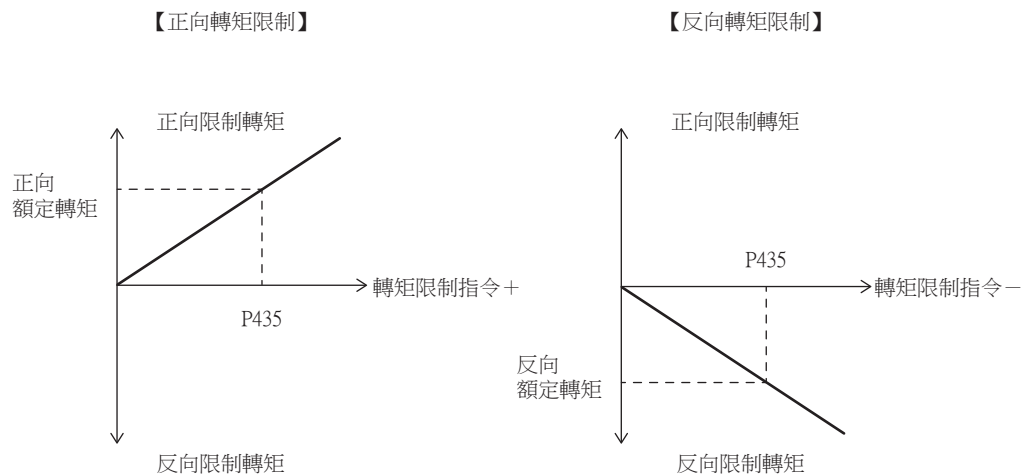
圖5-5 藉由類比轉矩指令的轉矩限制
