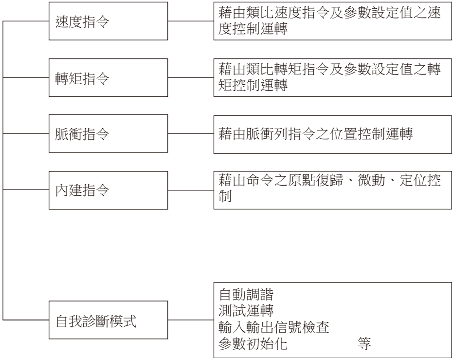
圖1-3 模式構成圖
