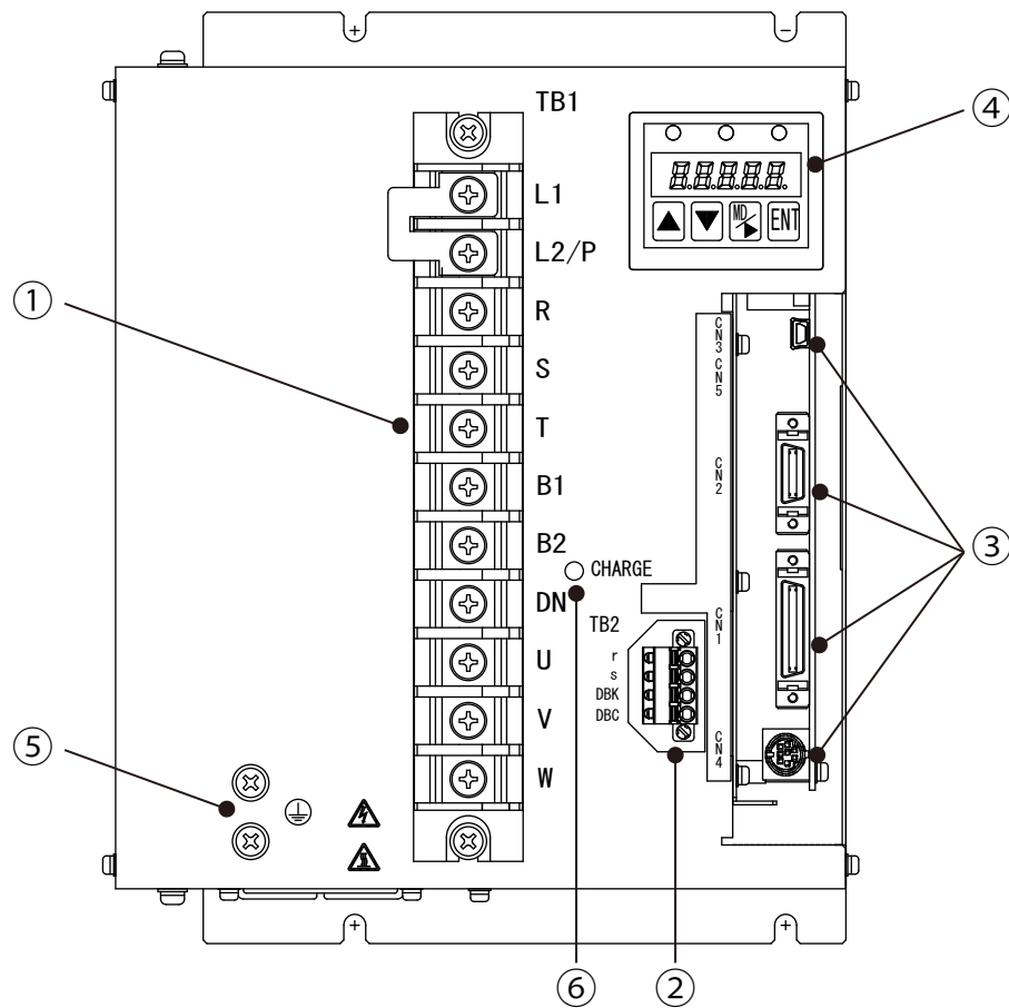
圖13-10 200V 7kW裝置本體正面圖（Type5）
