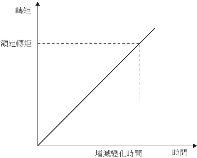
圖5-9 轉矩指令增減變化時間與額定轉矩的關係
