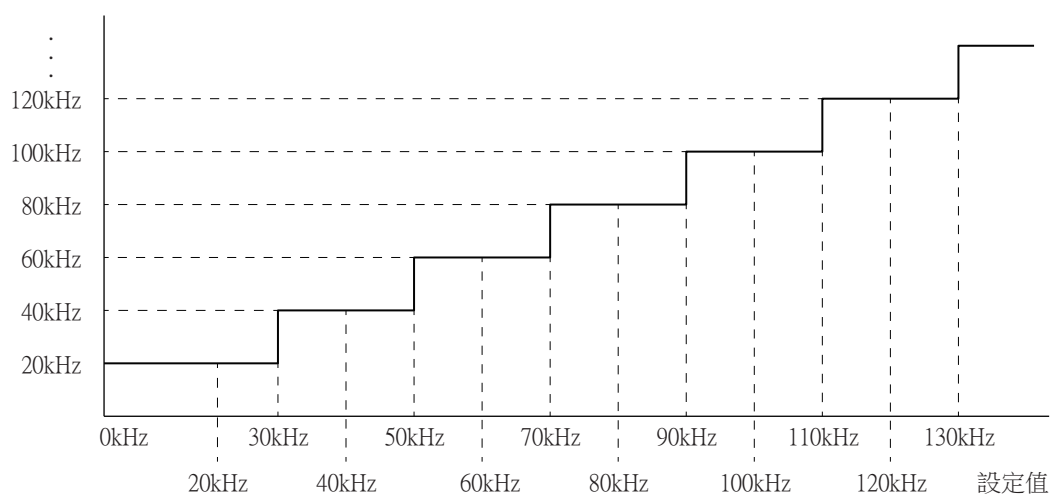
圖5-29 OUT POS輸出頻率
