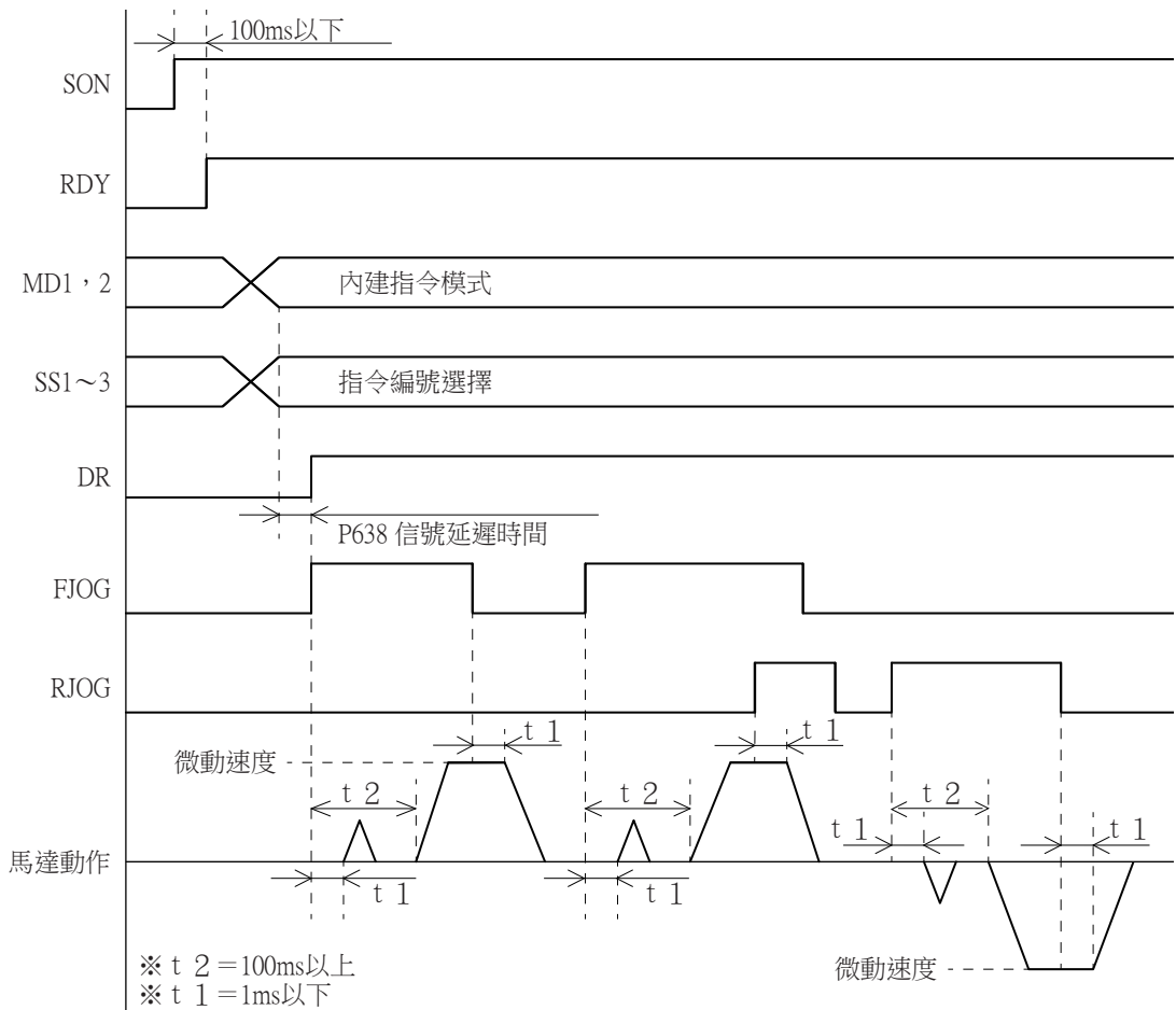
圖5-14 微動動作時序圖
