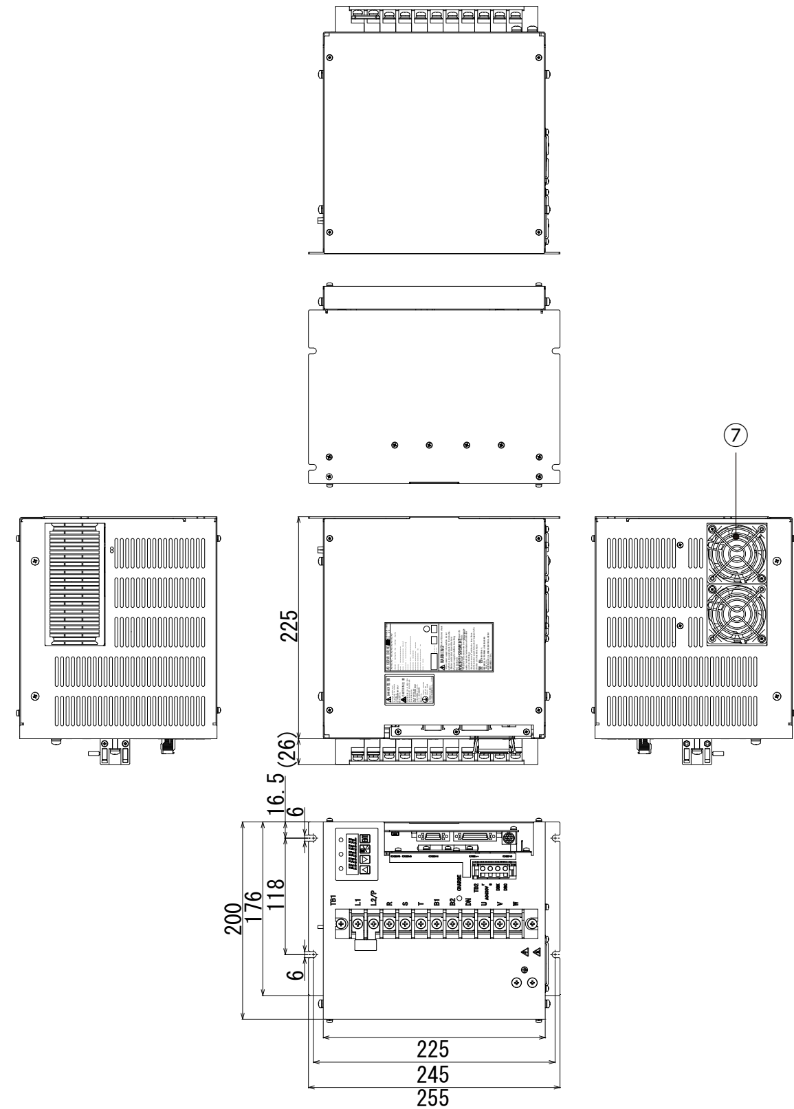
圖13-13 400V 7kW裝置本體外形圖 (Type7)
