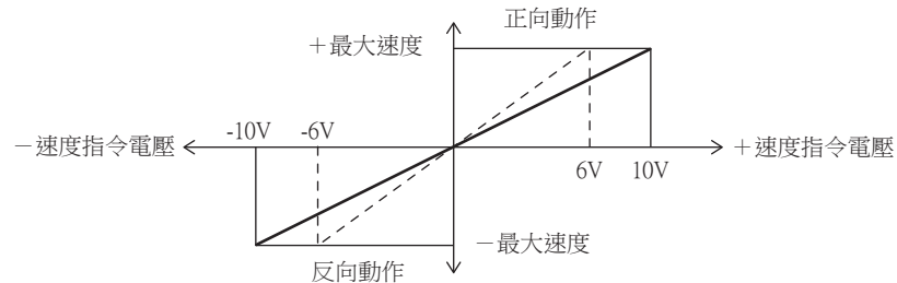
圖5-1 類比速度指令與馬達動作速度的關係
