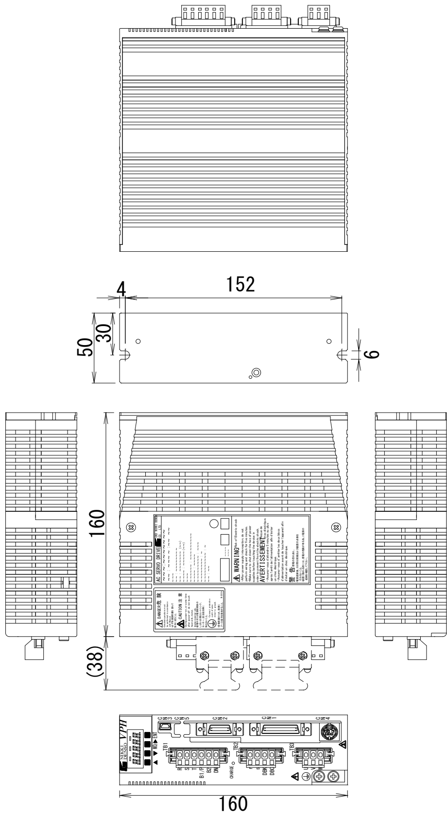
圖13-1 400W以下裝置本體外形圖（Type1）
