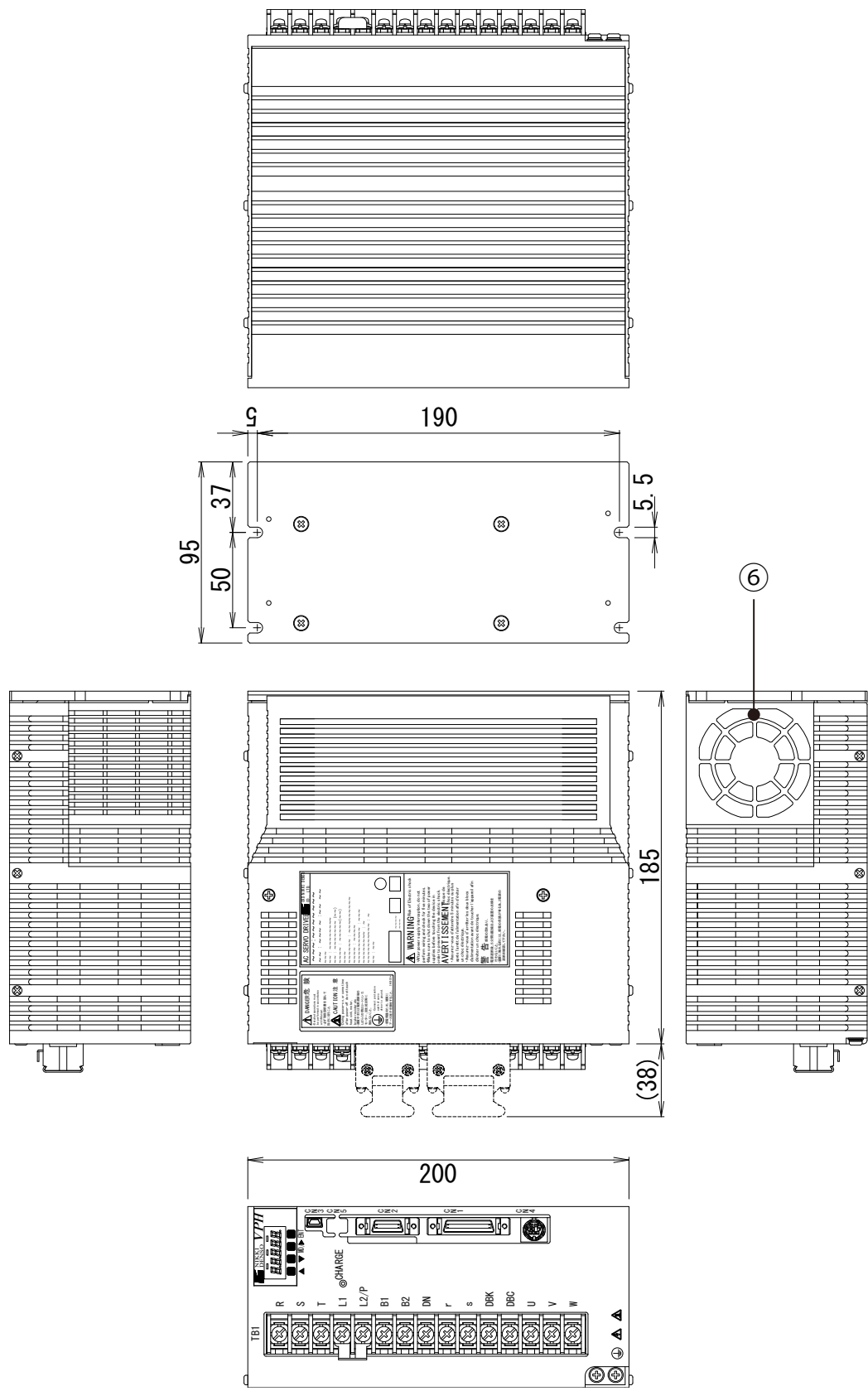
圖13-5 1.5kW、2.2kW裝置本體外形圖（Type3）
