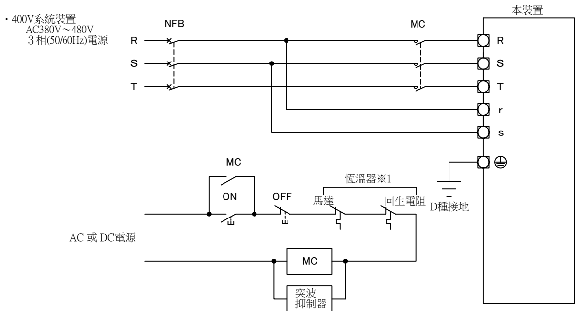
圖2-9 3相電源時具代表性的電源迴路(400V系統裝置)
