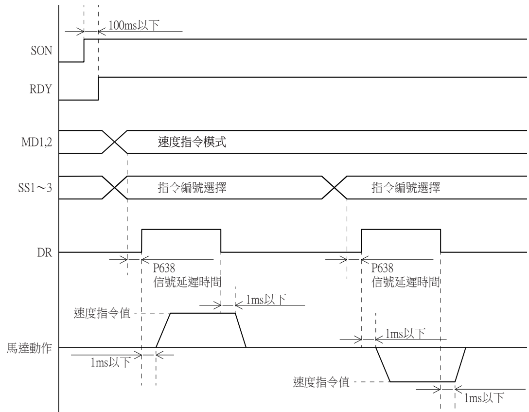
圖5-3 內部速度指令時序圖
