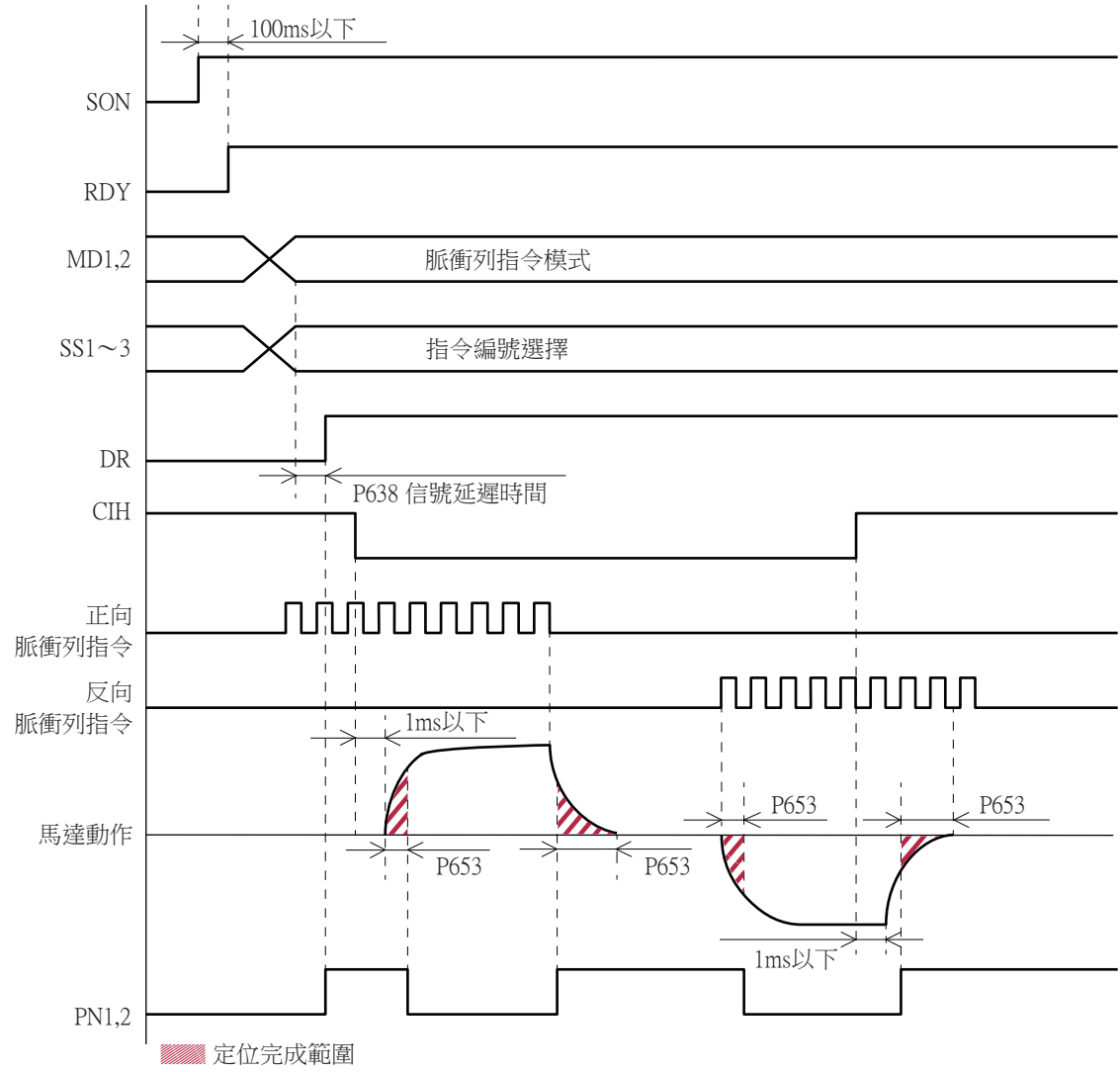
圖5-11 脈衝列指令時序圖
