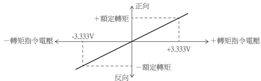
圖5-6 類比轉矩指令與馬達輸出轉矩的關係
