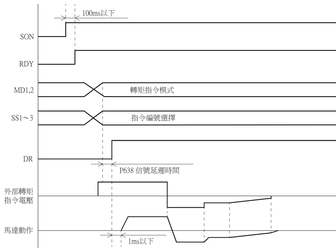
圖5-7 類比轉矩指令時序圖
