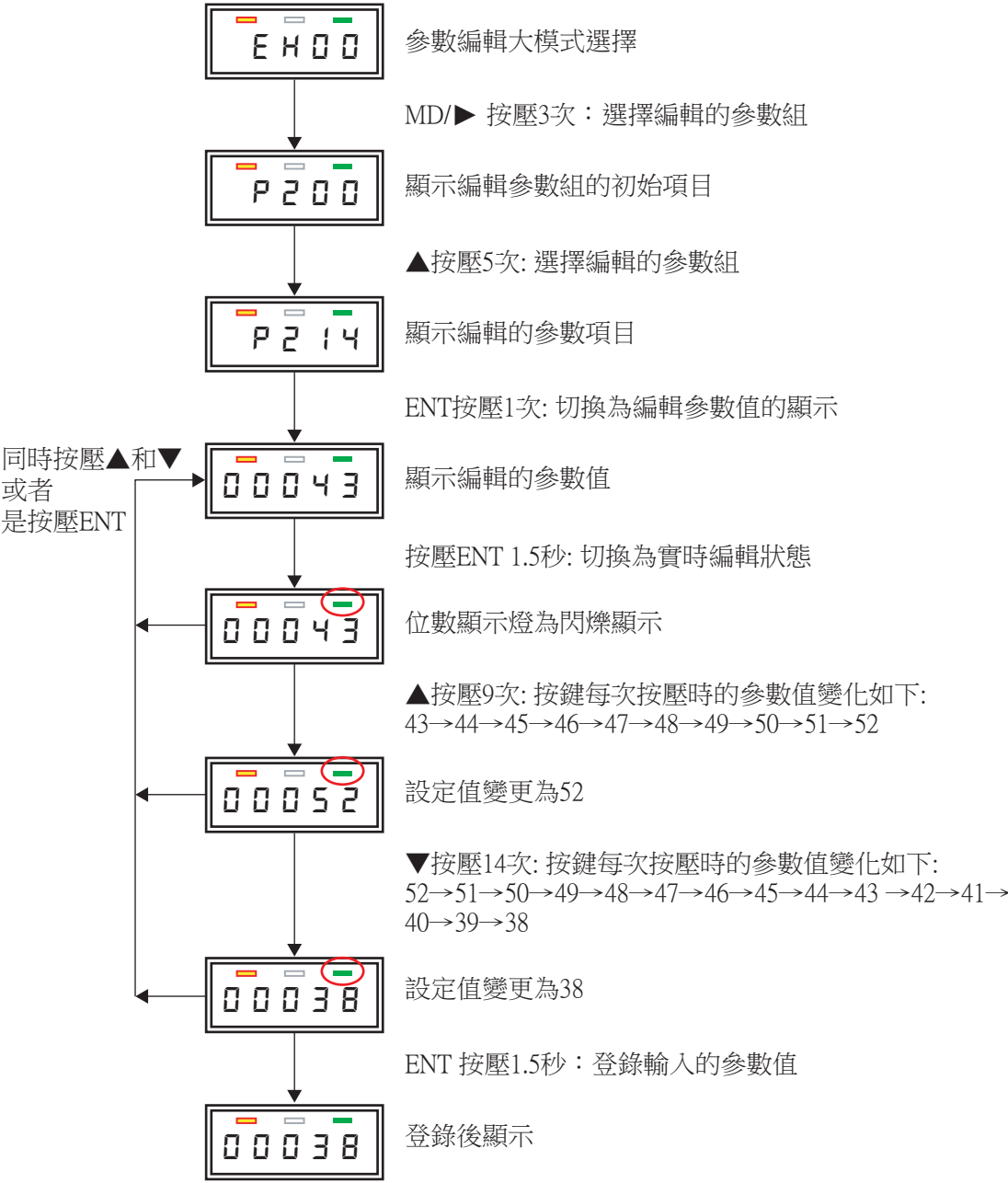
圖12-8 P214參數值(最大5位數): 依序變更為00043→00052→00038
