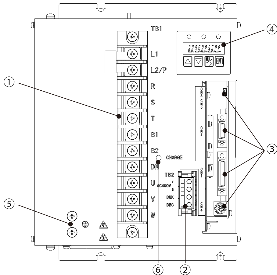
圖13-14 400V 7kW裝置本體正面圖（Type7）
