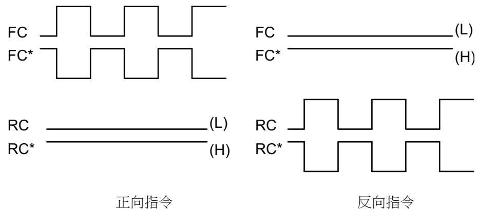
圖3-5 方向別脈衝
