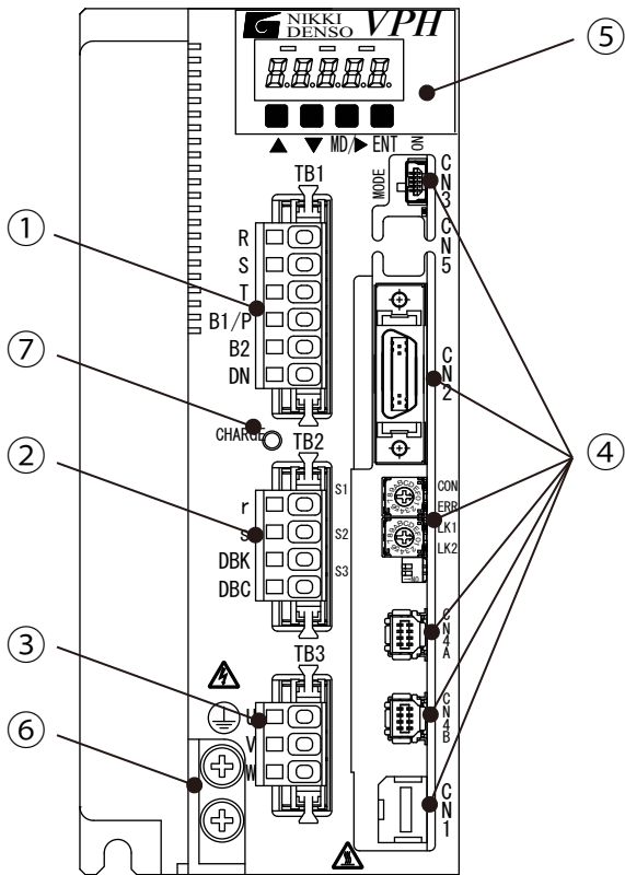
图13-4 800W驱动器主体正面图（Type2）
