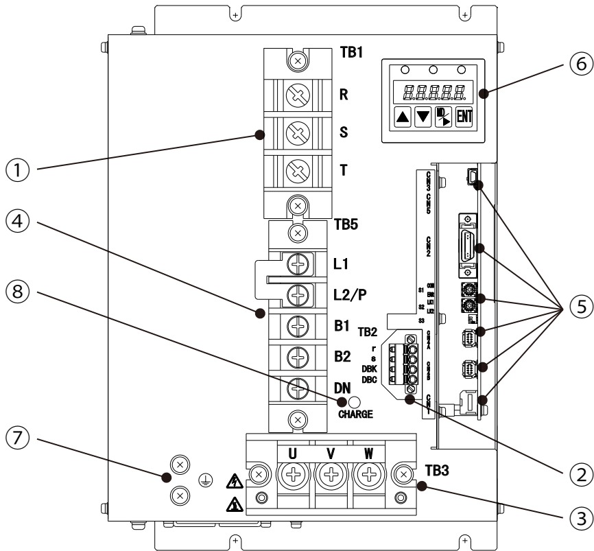
图13-12 15kW驱动器主体正面图（Type6）
