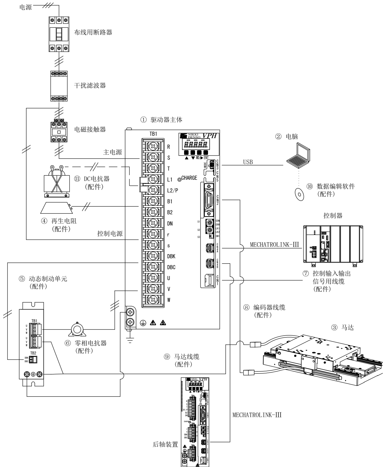
图1-2 1.5kW级以上VPH HE类型 系统构成
