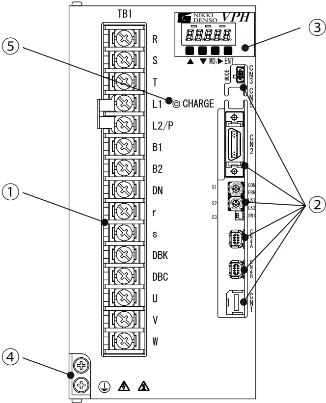
图13-6 1.5kW、2.2kW驱动器主体正面图（Type3）
