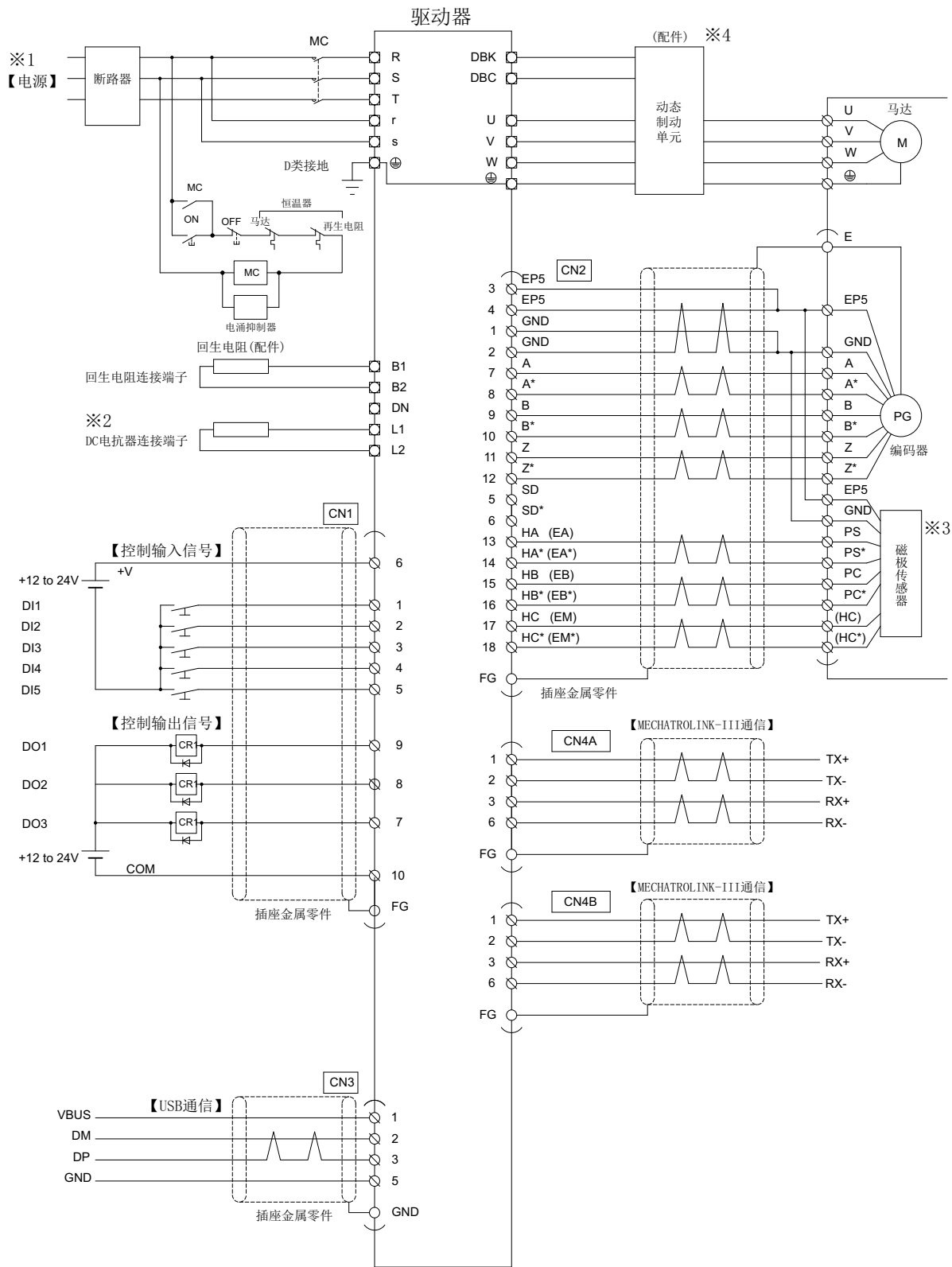
图3-1 外部连接图
