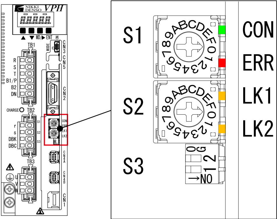
图1-4 通信状态显示LED外观
