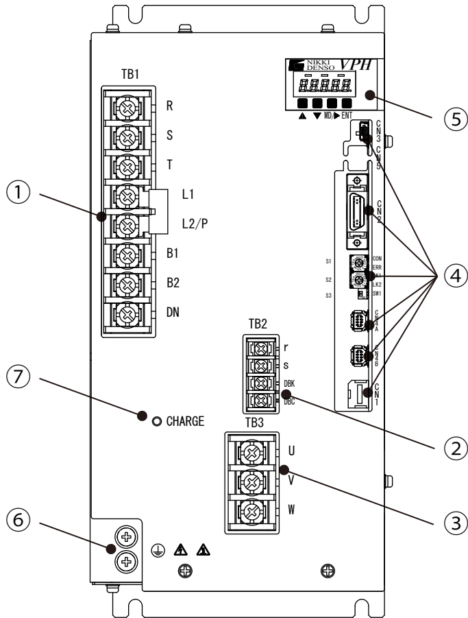
图13-8 3.3kW驱动器主体正面图（Type4）
