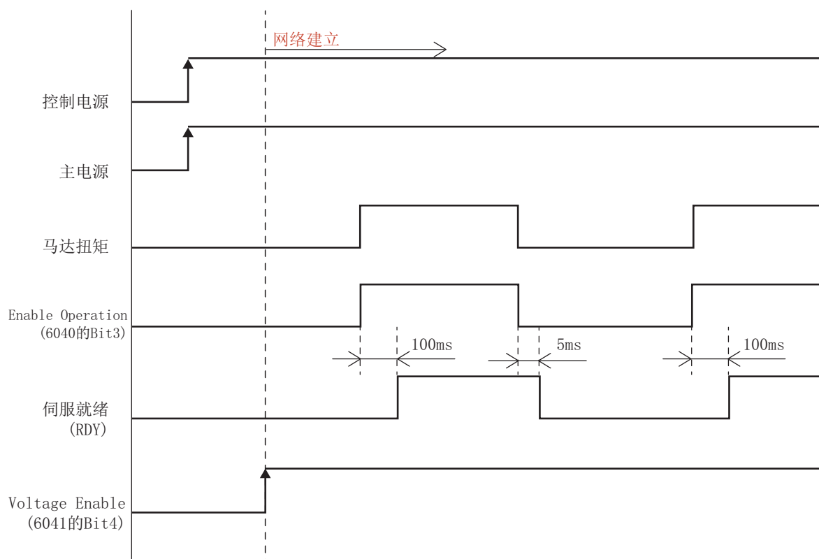
图2-10 时序图
