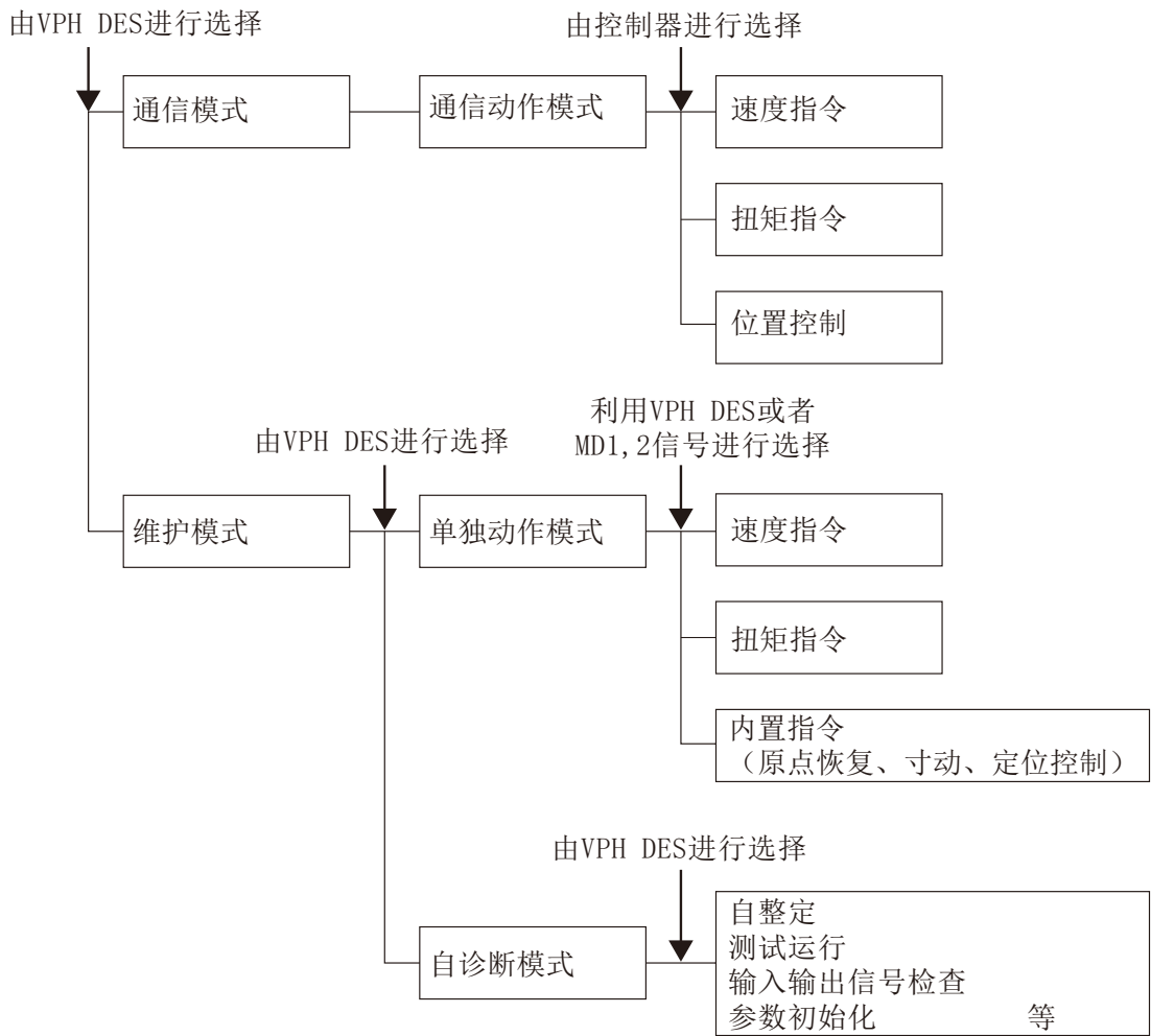
图1-5 模式构成图
