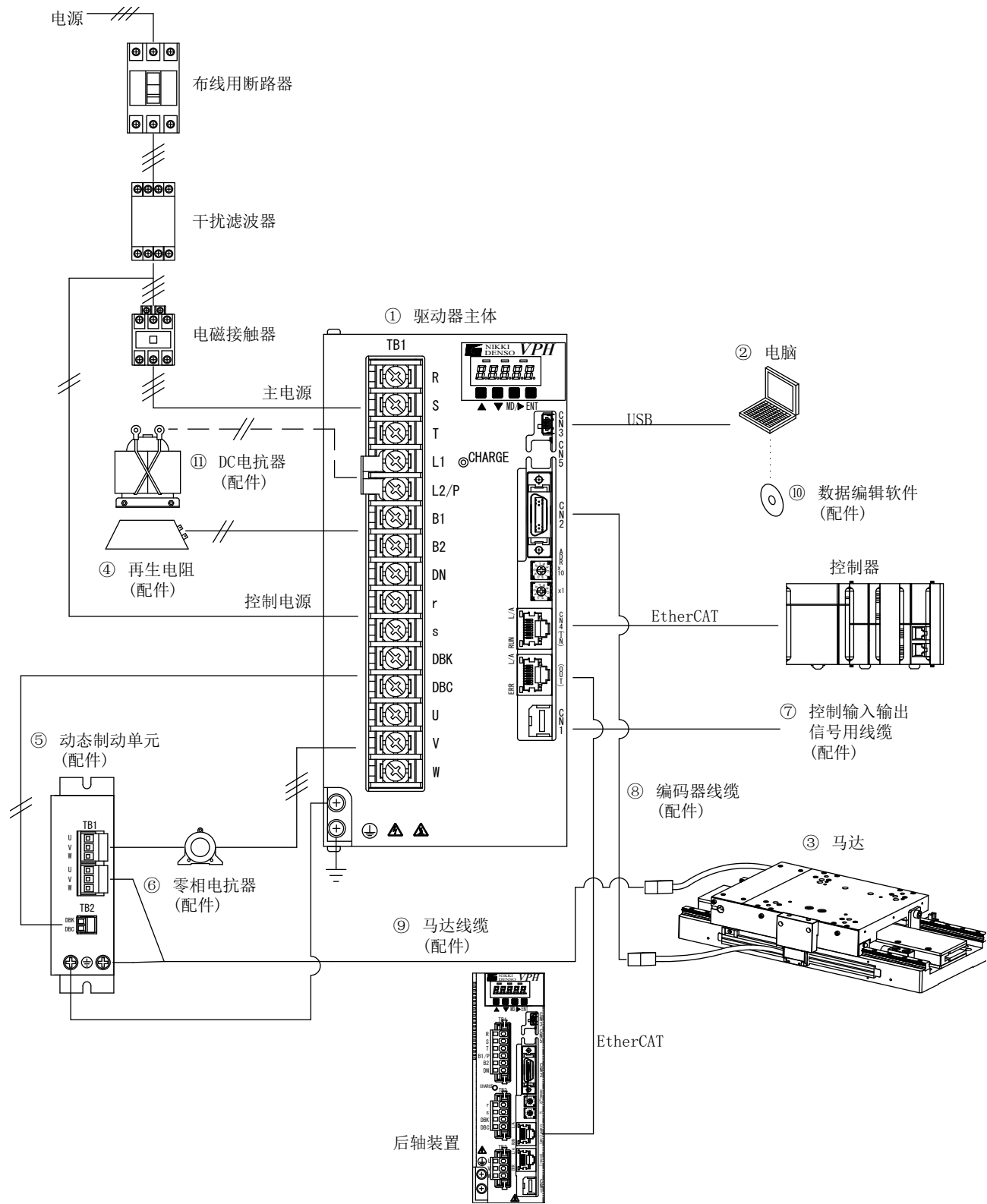
图1-2 1.5kW级以上VPH HD类型 系统构成
