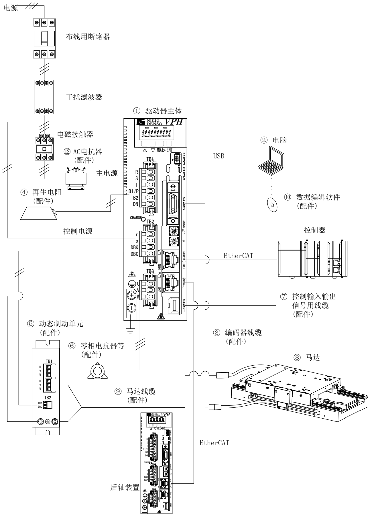
图1-1 800W级以下VPH HD类型 系统构成
