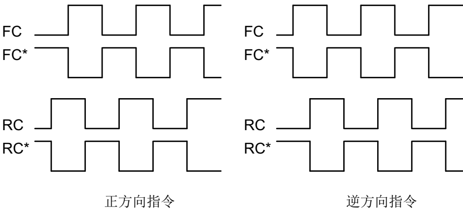
图3-3 90° 相位差信号
