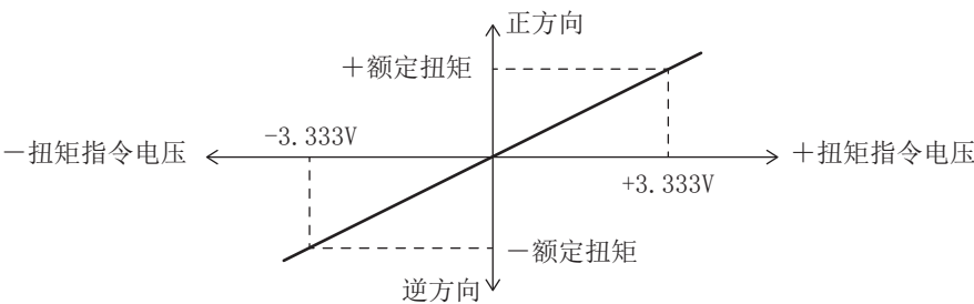
图5-6 模拟扭矩指令与马达输出扭矩的关系
