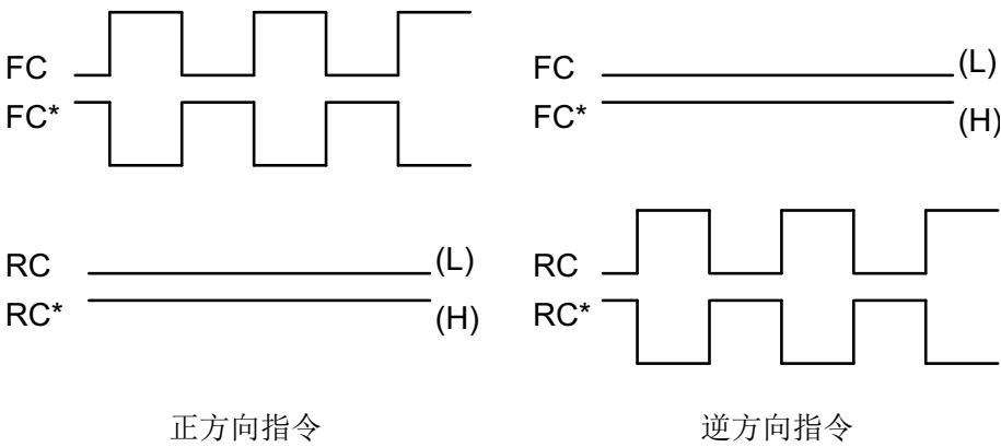
图3-5 各方向的脉冲
