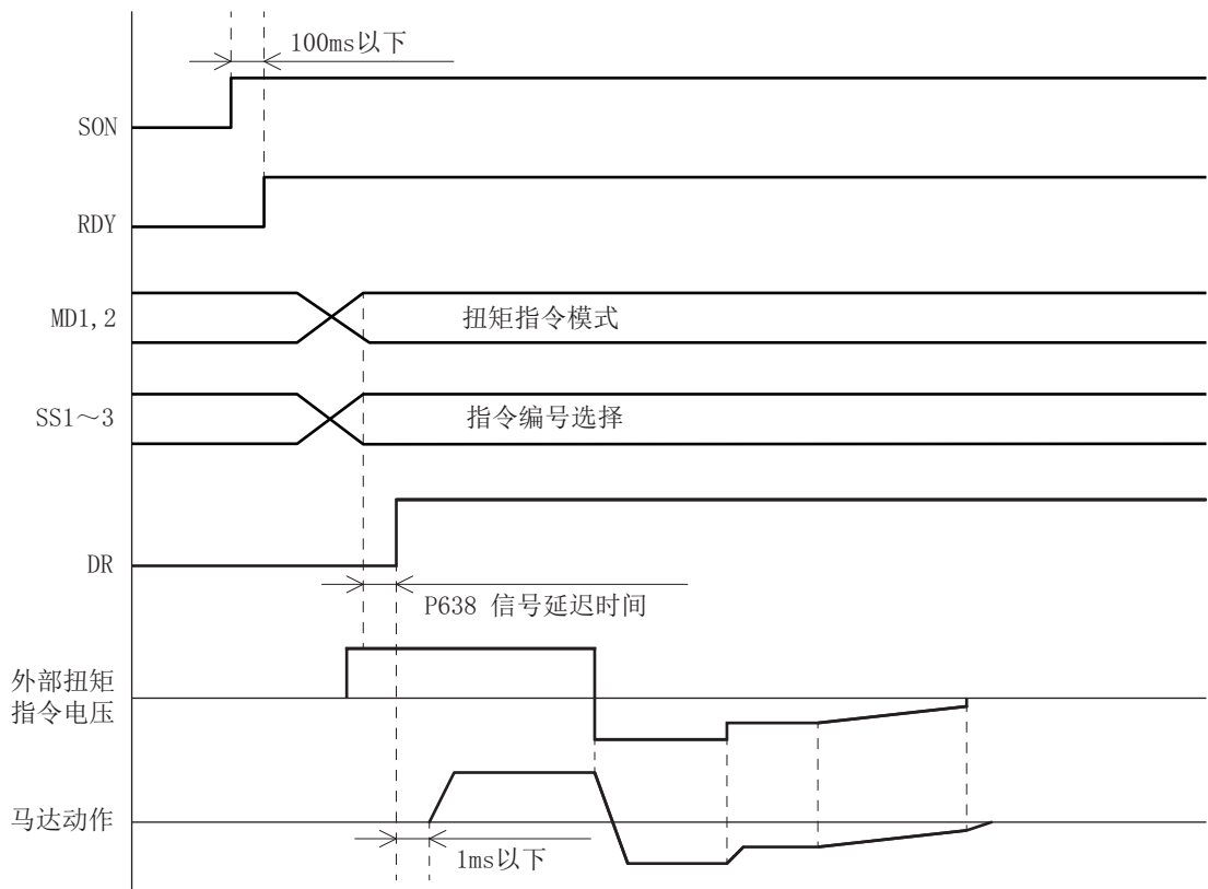
图5-7 模拟扭矩指令时序图
