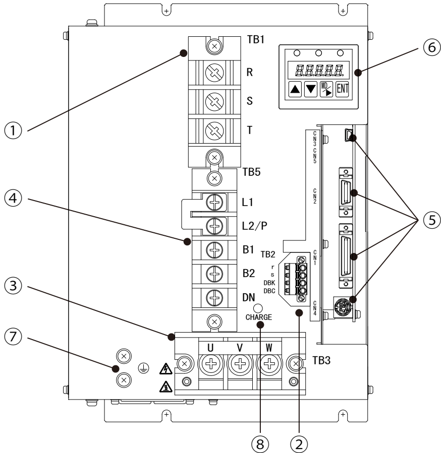
图13-12 15kW驱动器主体正面图（Type6）
