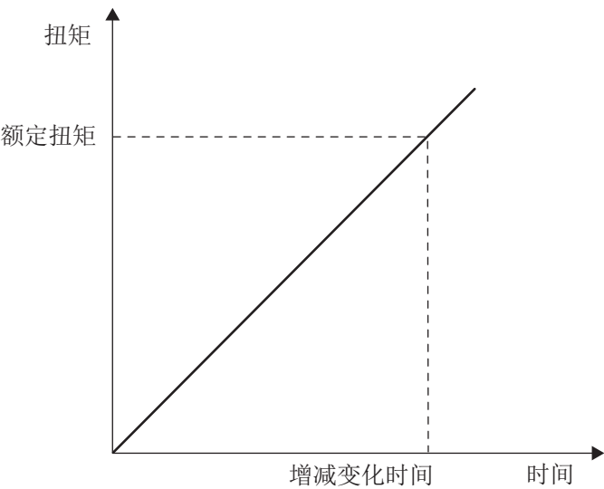
图5-9 扭矩指令增减变化时间的关系
