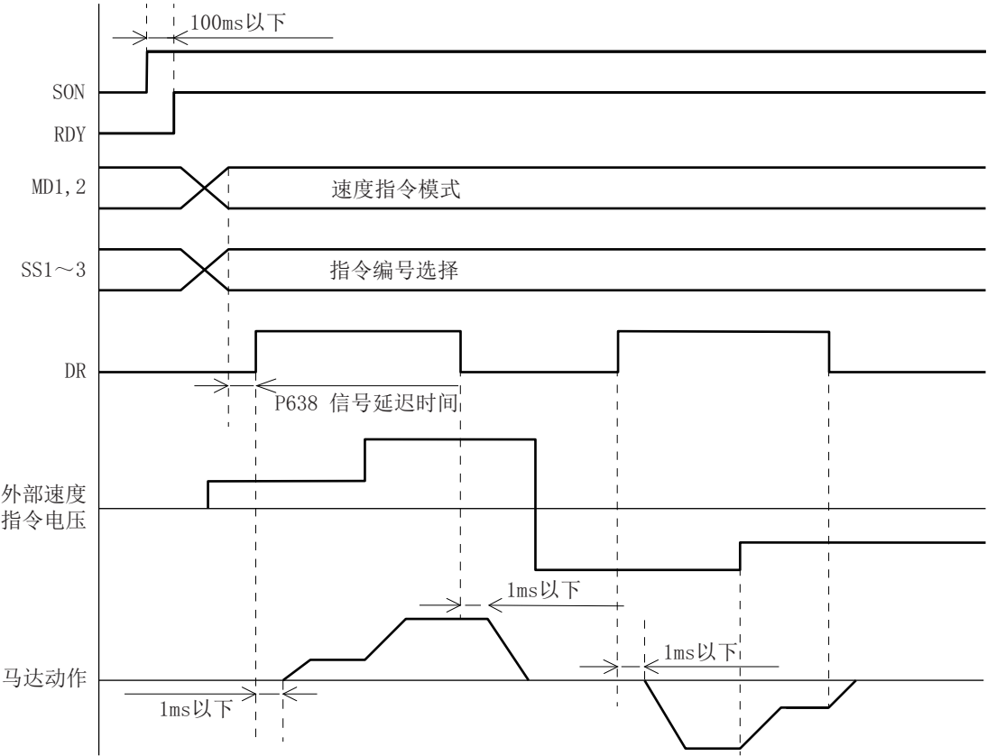
图5-2 模拟速度指令时序图
