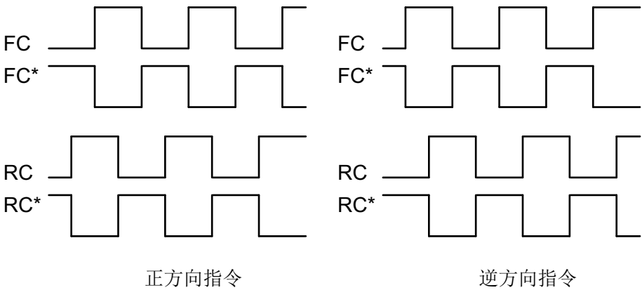
图3-4 90° 相位差信号
