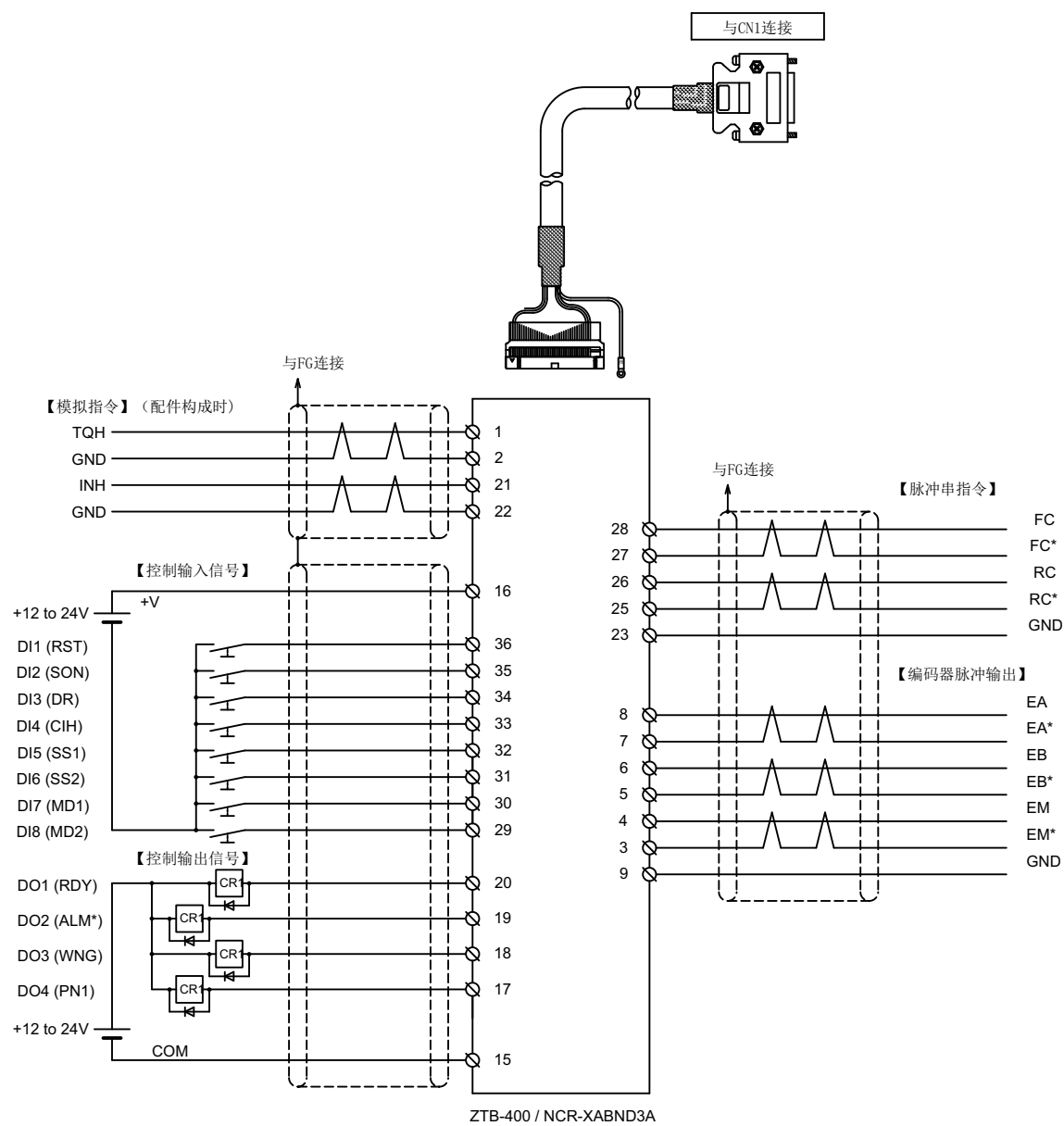
图3-3 I / O端子台（配件）连接图
