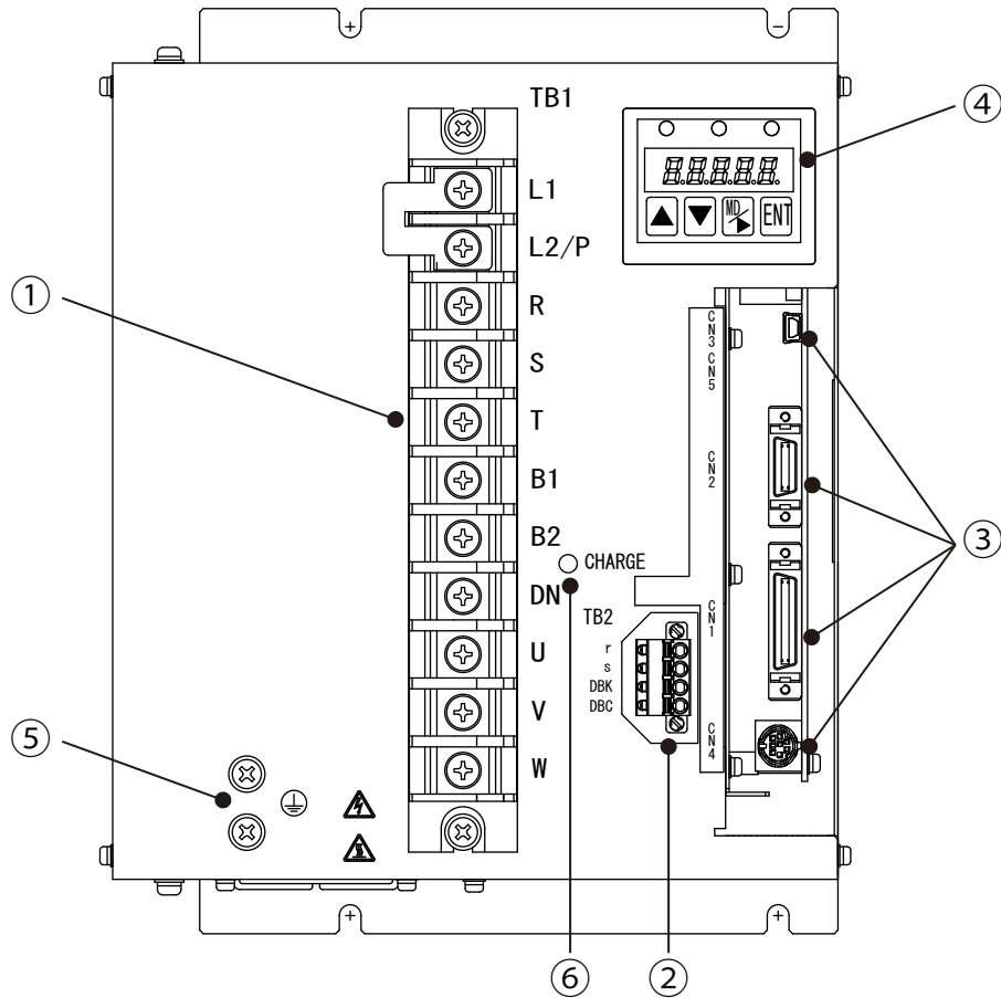
图13-10 200V 7kW驱动器主体正面图（Type5）
