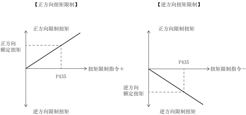
图5-5 基于模拟扭矩指令的扭矩限制
