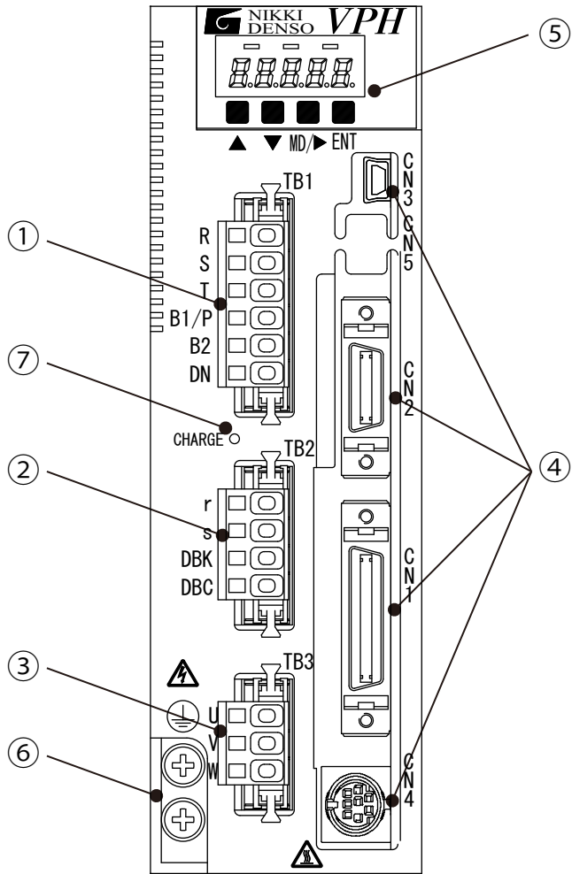
图13-2 400W以下的驱动器主体正面图（Type1）
