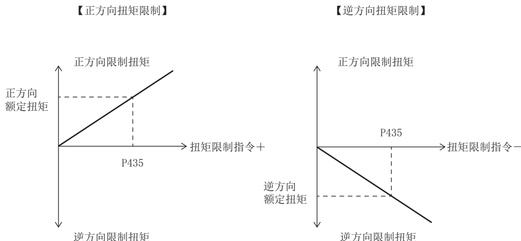
图5-13 基于模拟扭矩指令的扭矩限制
