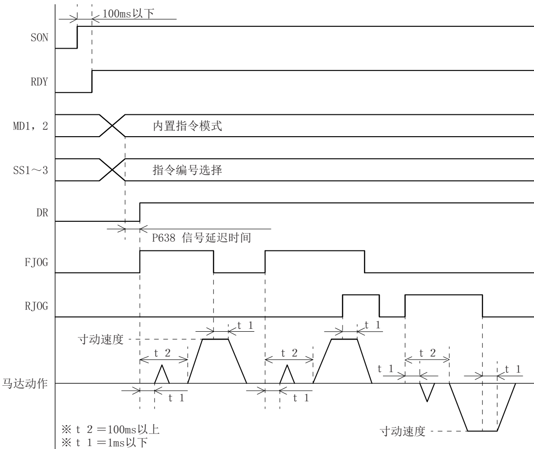
图5-14 寸动动作时序图
