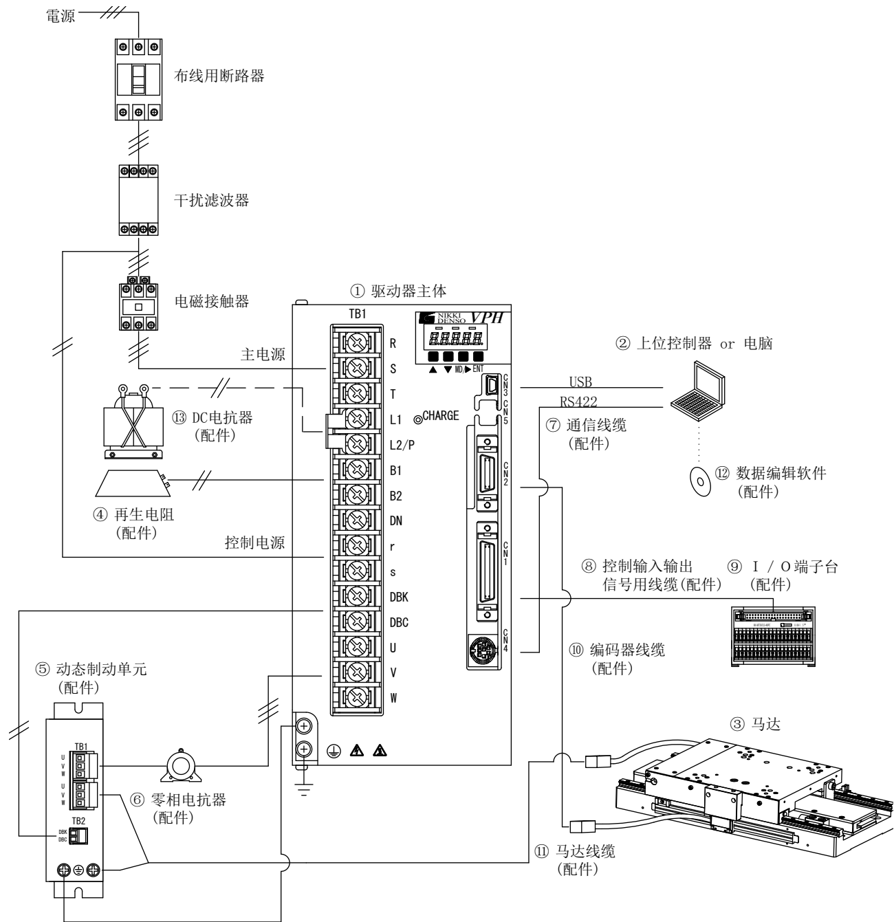
图1-2 1.5kW级以上VPH HA类型 系统构成
