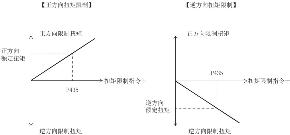
图5-17 基于模拟扭矩指令的扭矩限制
