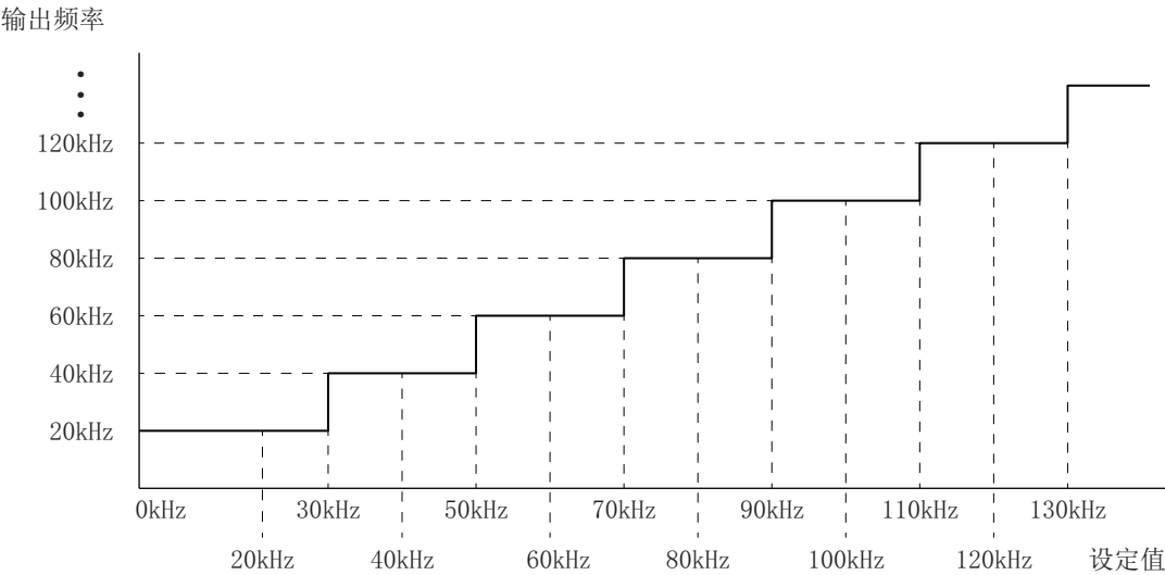
图 5-29 OUT POS 输出频率
