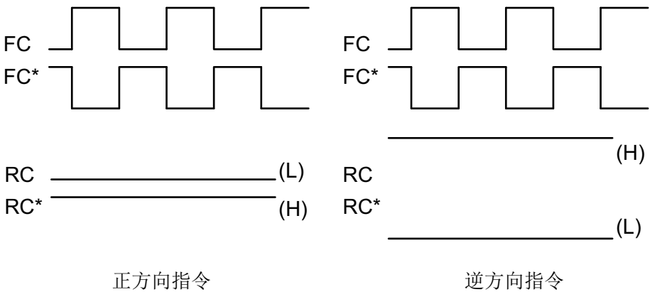
图3-6 方向信号 + 传送脉冲
