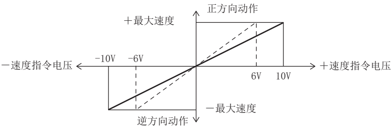
图5-1 模拟速度指令与马达动作速度的关系
