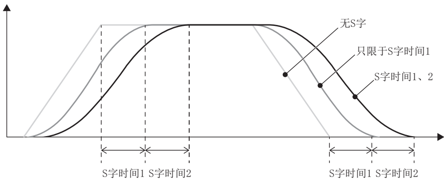
图5-12 S字加减速动作例
