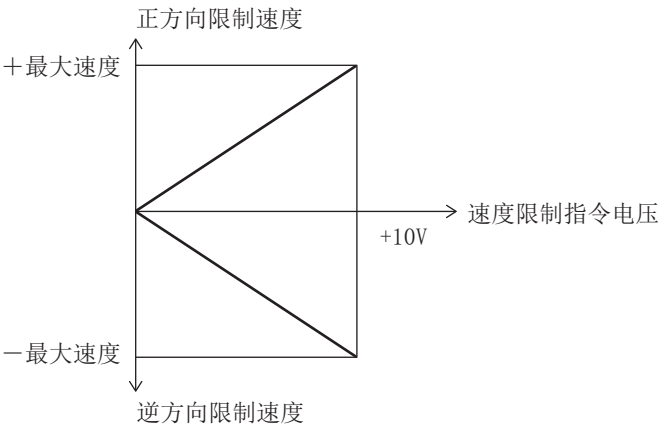
图5-10 基于模拟速度指令的速度限制
