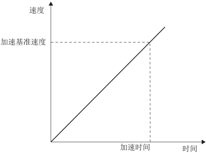
图5-4 速度指令模式时的加速基准速度和加速时间的关系
