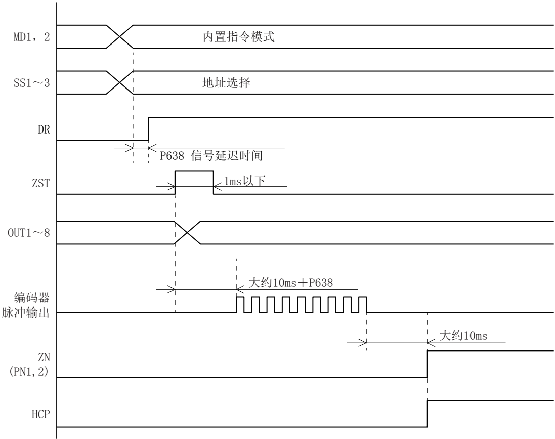
图5-30 OUT POS 时序图
