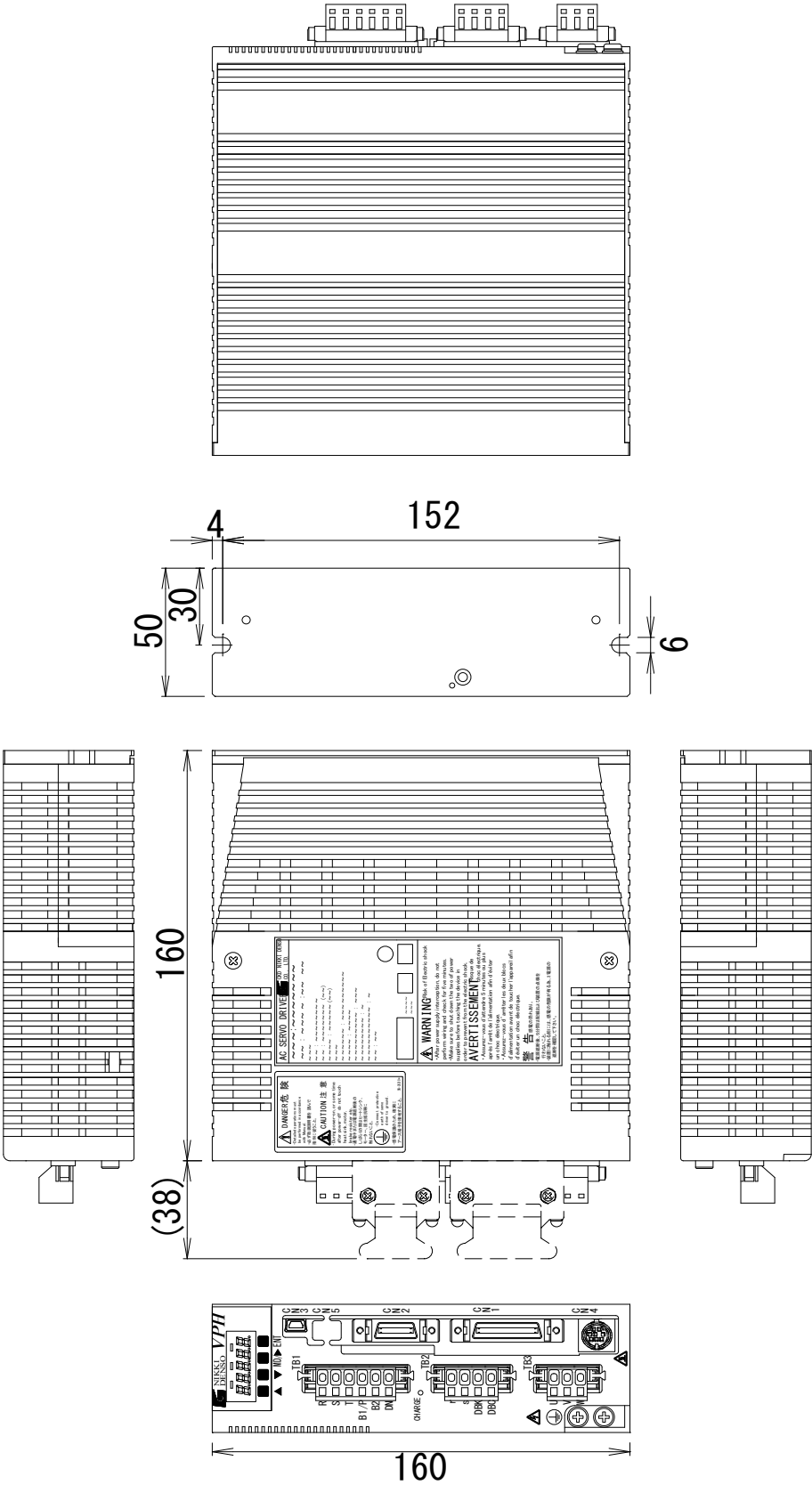
图13-1 400W以下驱动器主体外形图 (Type1)
