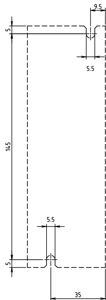
取付穴位置
