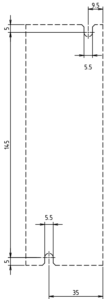
取付穴位置
