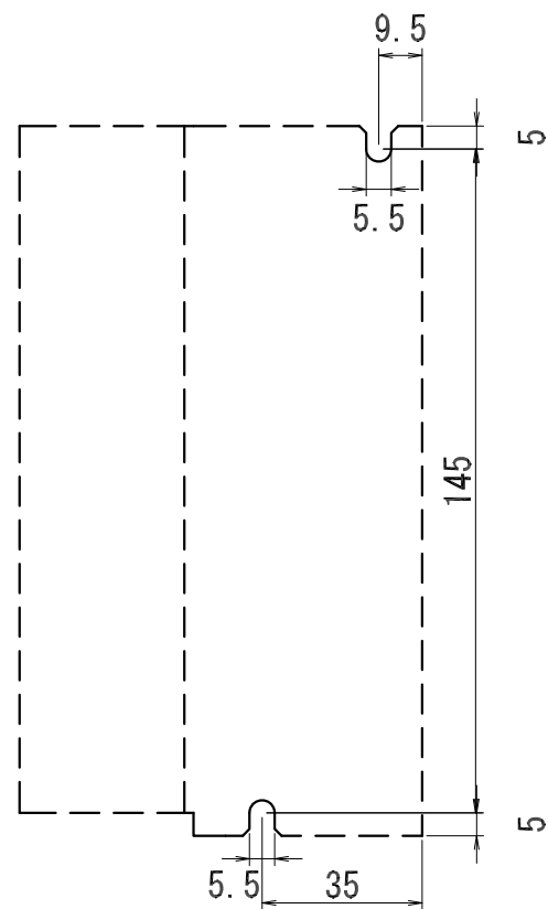
取付穴位置
