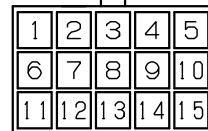
センサ・エンコーダコネクタ 型式: 172171-1(ハウジング) 170363-1(ケーブル)
