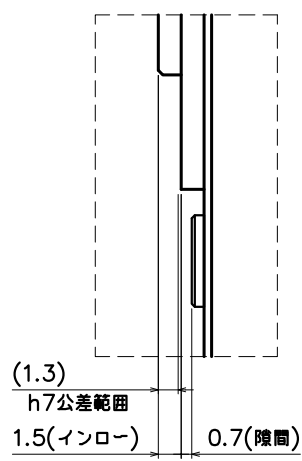
”A”部詳細 (S=3/1)
